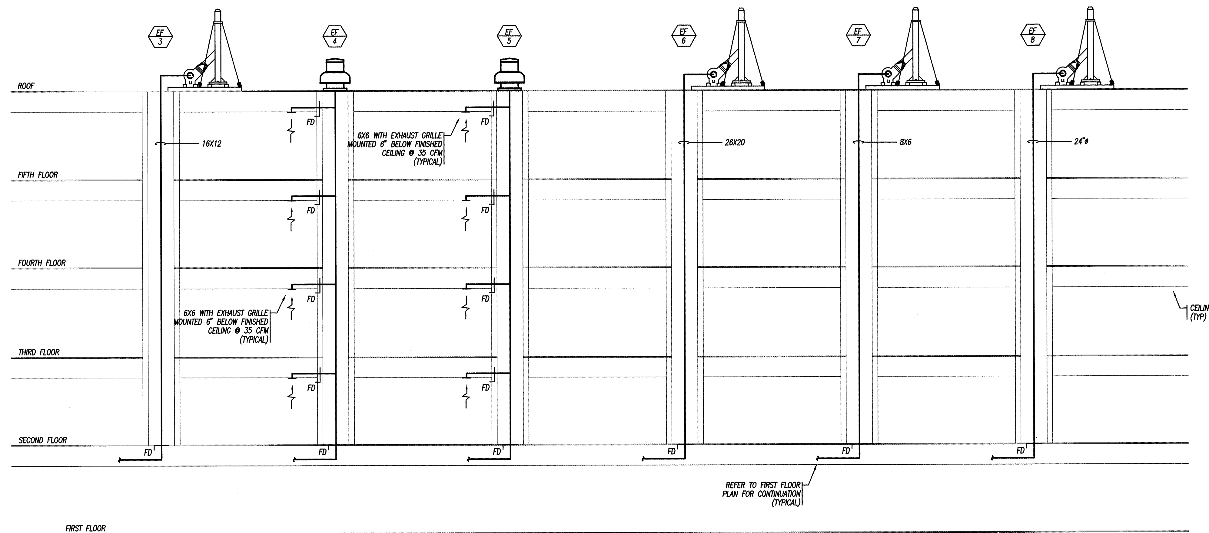
RESTROOM EXHAUST RISER FAN EF-3
