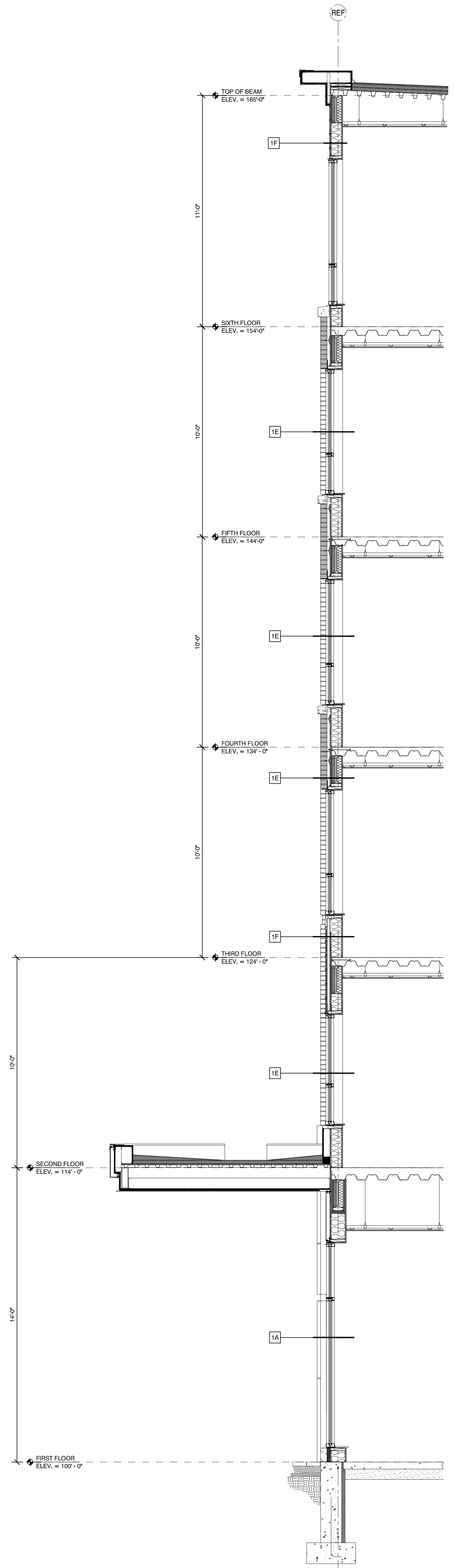
7 WALL SECTION SCALE: 3/8" = 1'-0"
