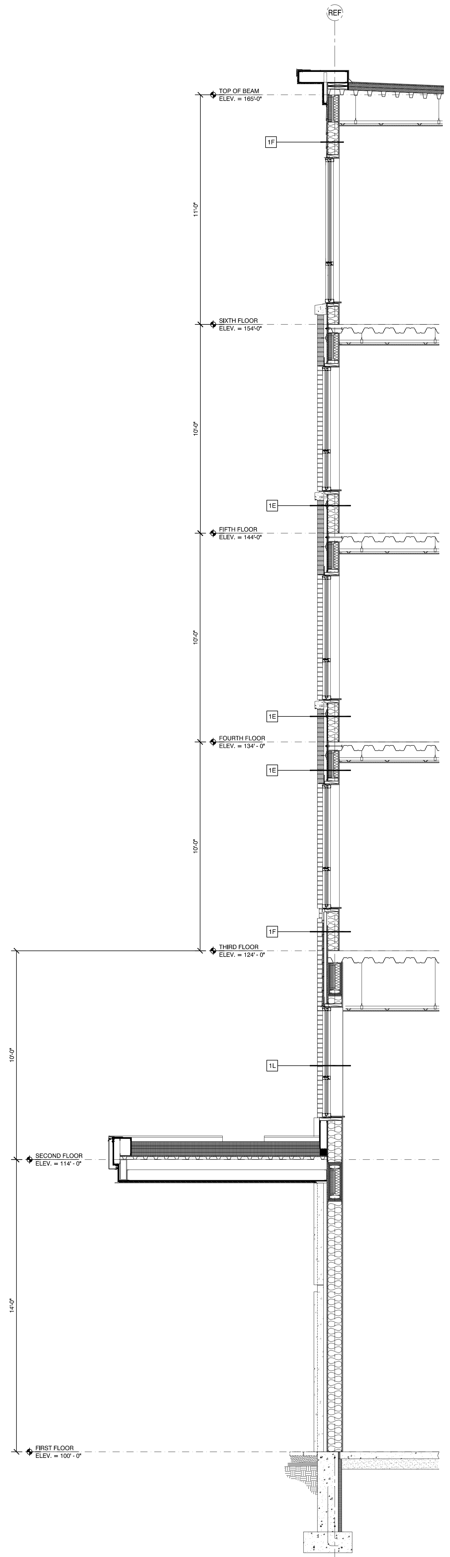
4 WALL SECTION SCALE: 3/8" = 1'-0"
