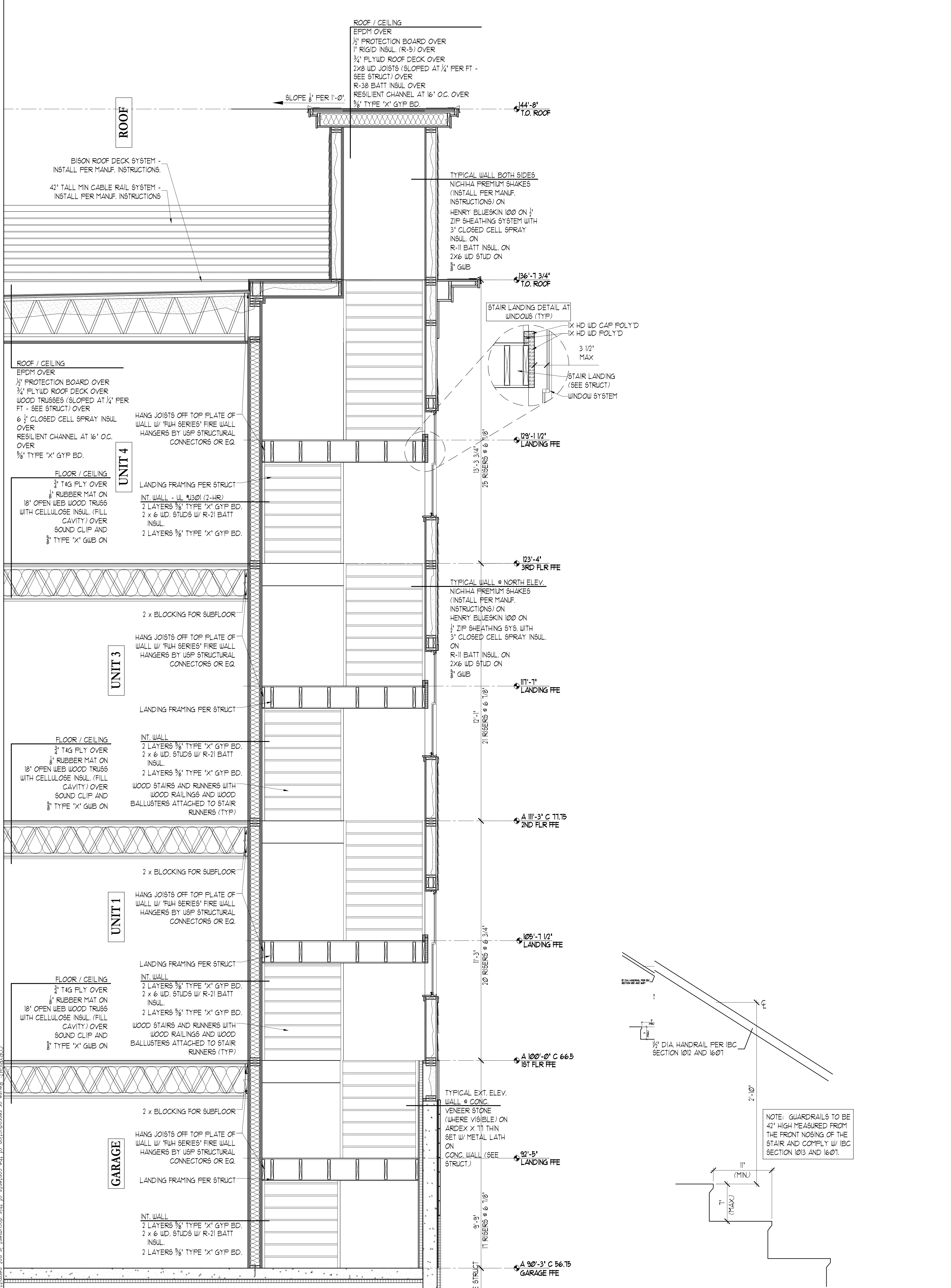
2 STAIR SECTION SCALE: 1/2" = 1'-0"
