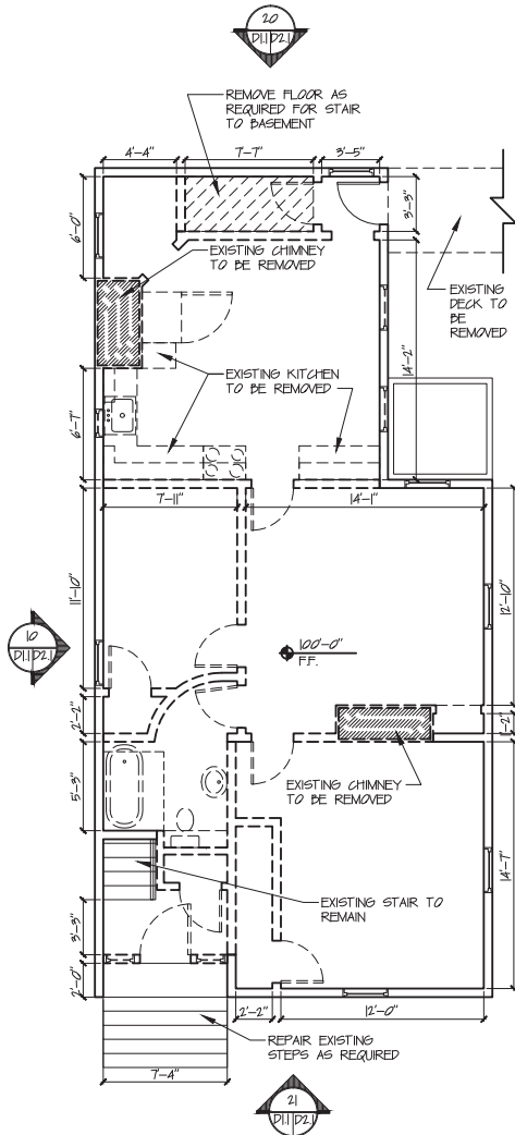
30 FIRST FLOOR SCALE: 1/8" = 1'-0"
