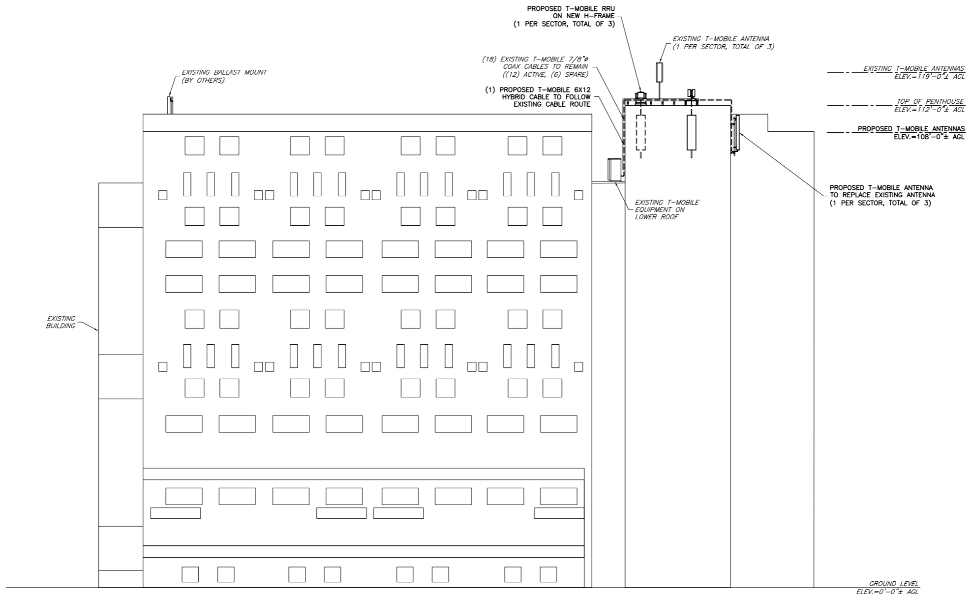
1 ELEVATION C-2 SCALE: 1" = 10'
