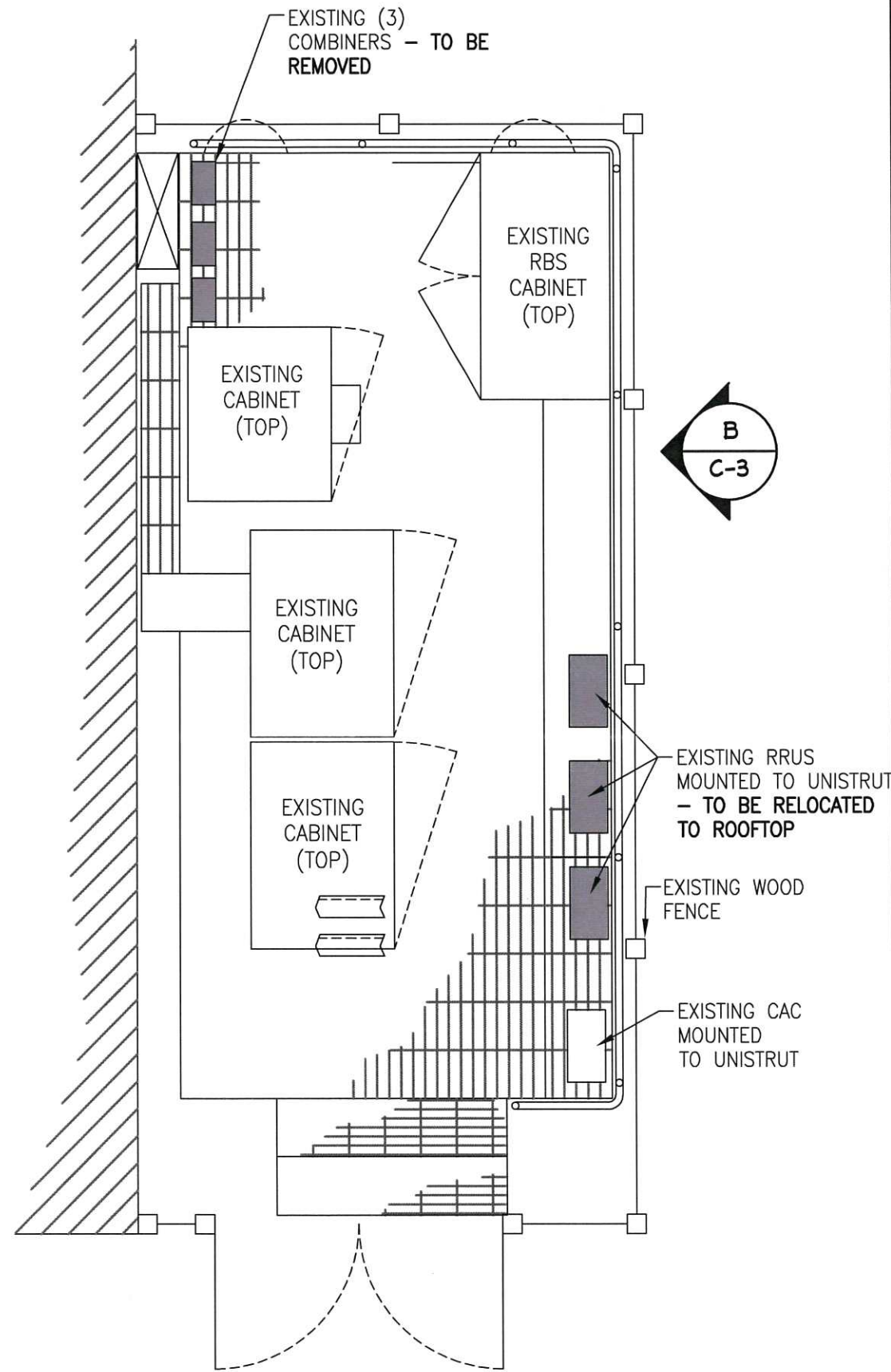
EQUIPMENT LAYOUT SCALE: N.T.S.
