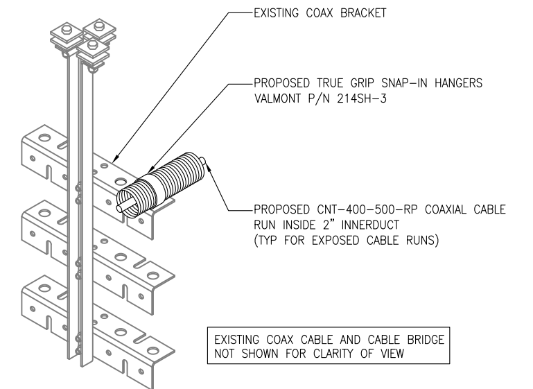
3 HOR. INNERDUCT/COAX DETAIL G-1 SCALE: N.T.S.
