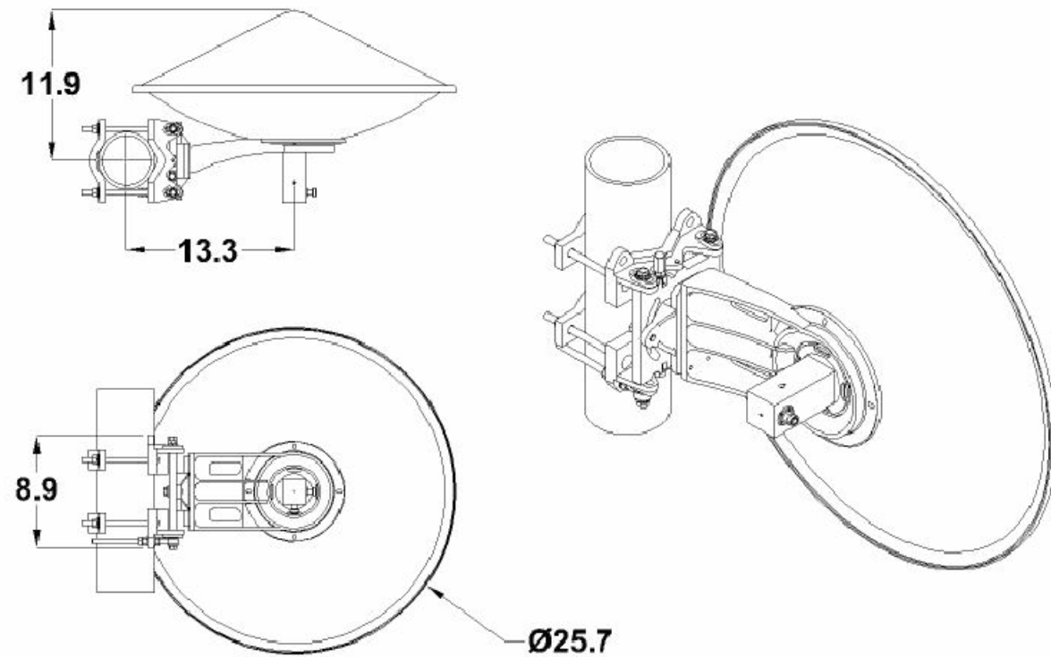
1 MICROWAVE DETAILS SCALE: N.T.S.
