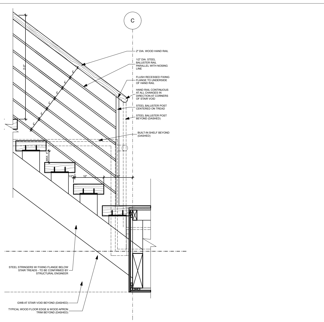
13 STAIR BALUSTRADE SCALE: 3/4" = 1'-0"
