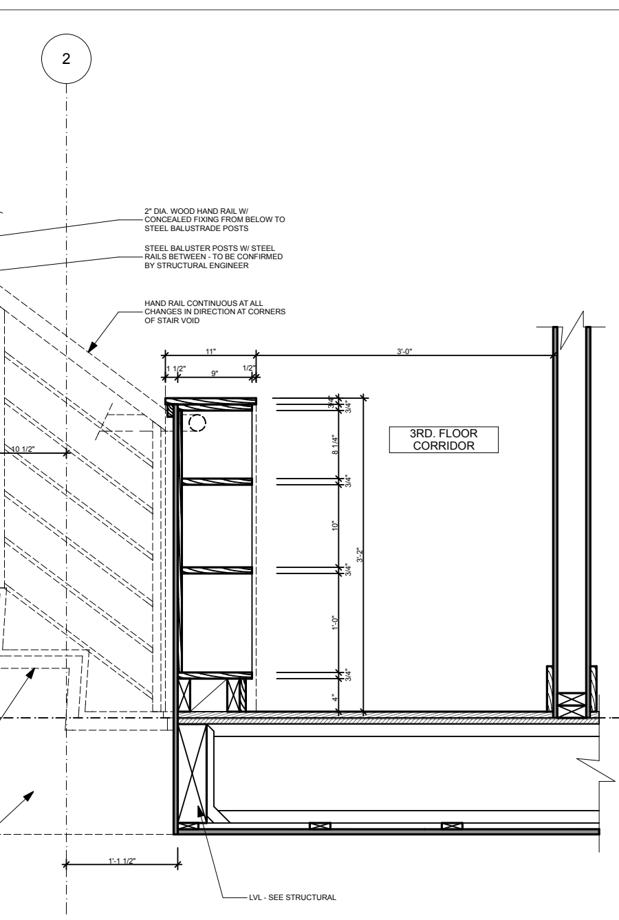
13 STAIR BALUSTRADE SCALE: 3/4" = 1'-0"
