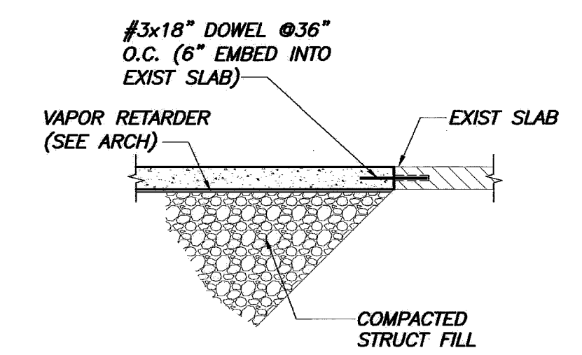
TYP SLAB INFILL DETAIL N.T.S.
