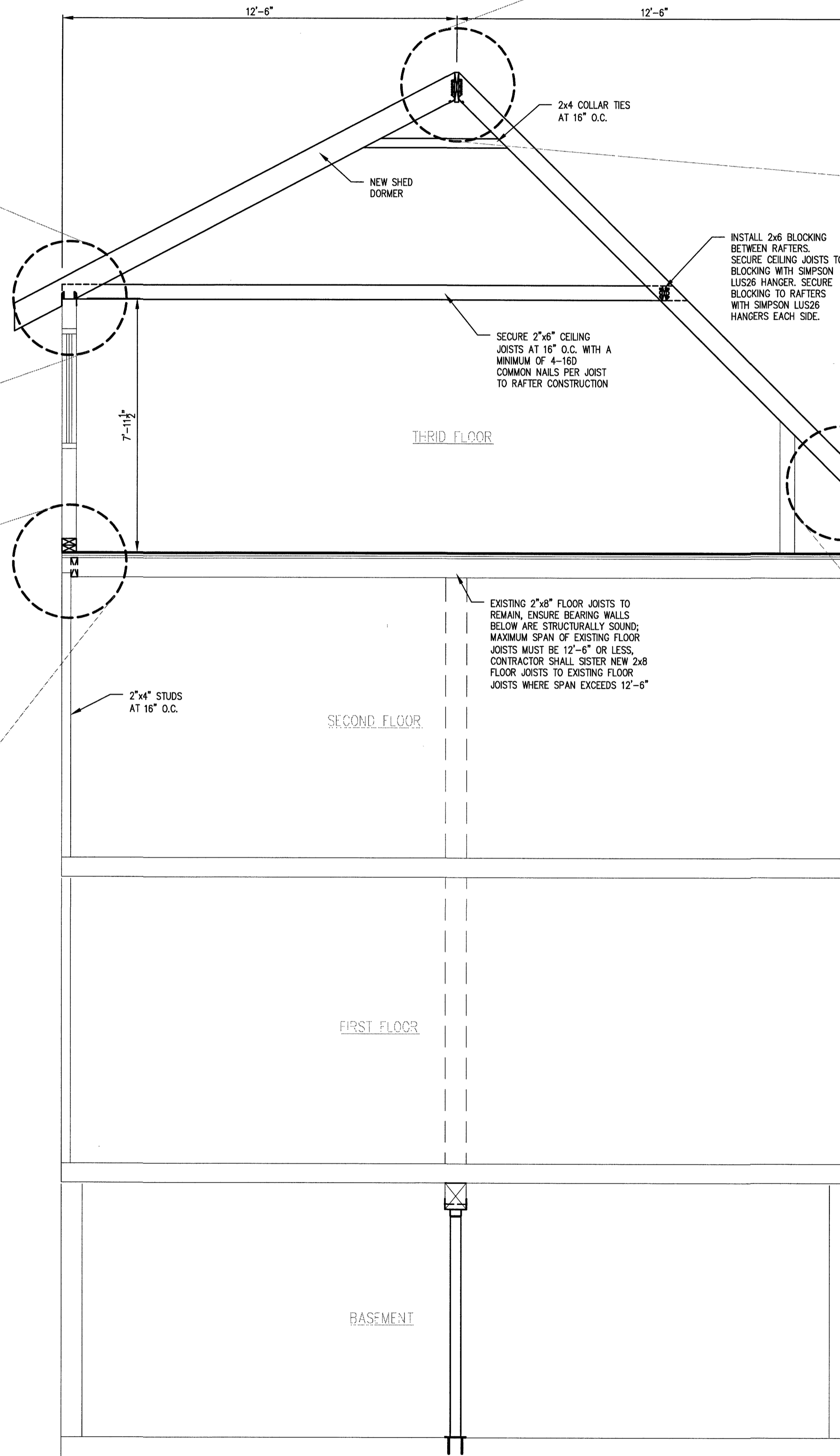
SECTION VIEW (A-A) SCALE: 3/8" = 1'-0"
