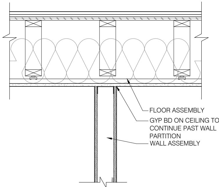
6 PARTITION DETAIL SCALE: 1" = 1'-0"
