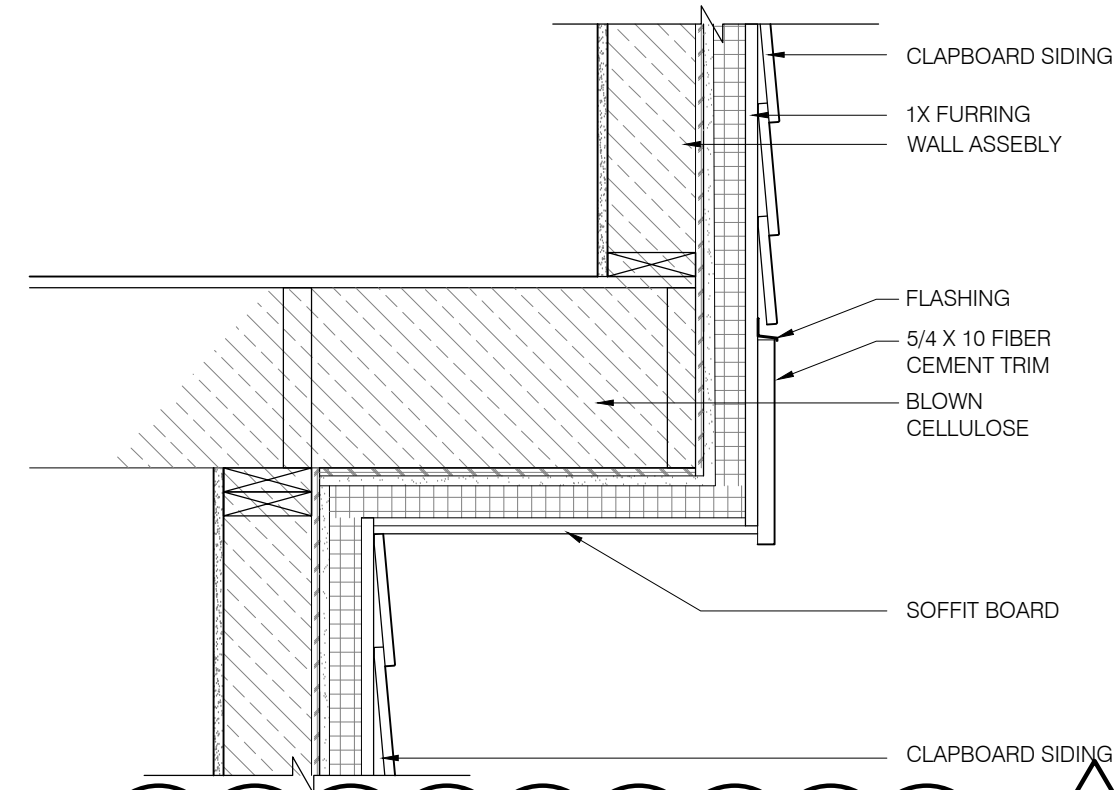
8 OVERHANG DETAIL SCALE: 1" = 1'-0"
