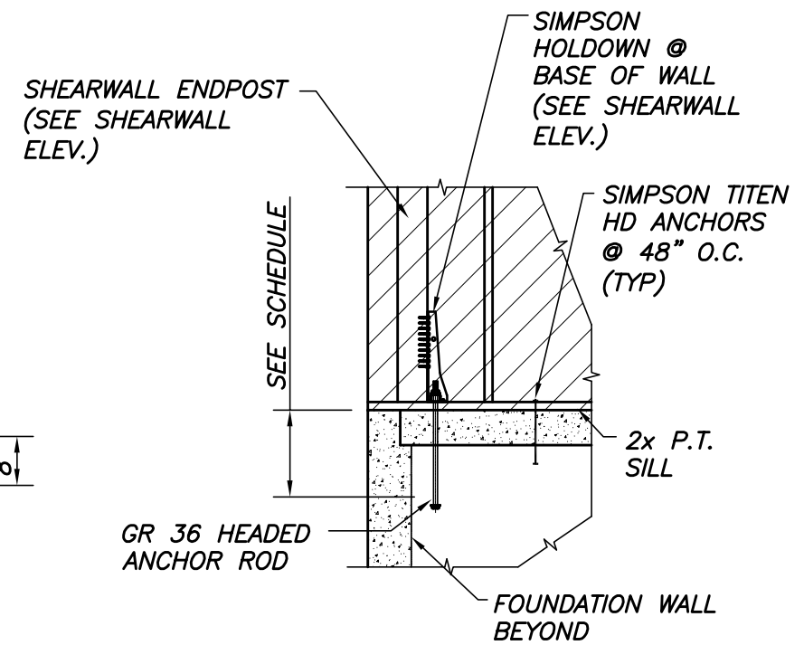
TYP HOLDOWN DETAIL N.T.S.
