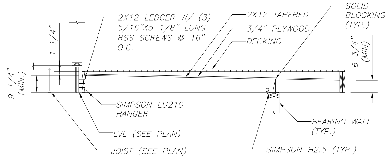
DECK DETAIL N.T.S.
