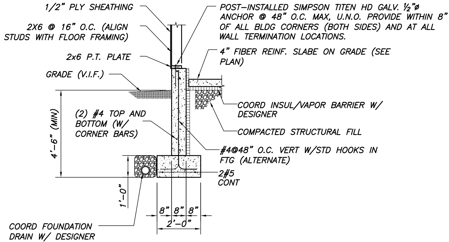
TYP FOUNDATION DETAIL N.T.S.
