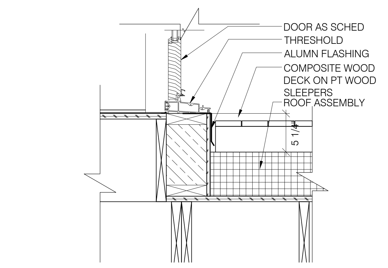
8 SILL - ROOFTOP DOOR SCALE: 1-1/2" = 1'-0"
