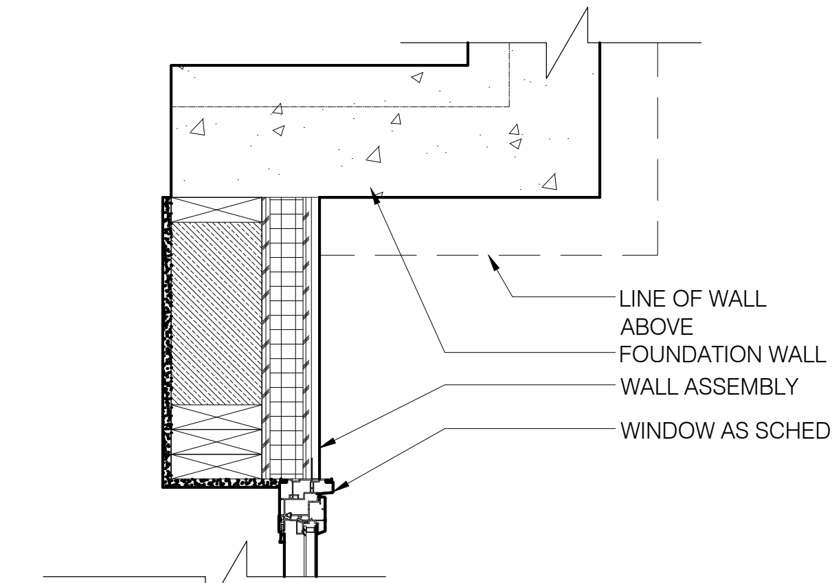
9 JAMB - FRONT SIDE LIGHTS SCALE: 1-1/2" = 1'-0"
