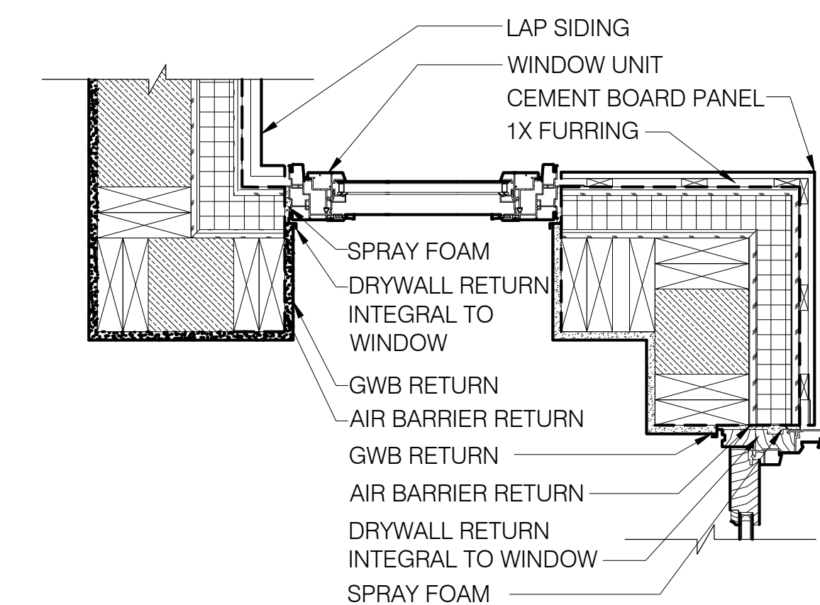
4 JAMB - BAY WINDOW SCALE: 1-1/2" = 1'-0"
