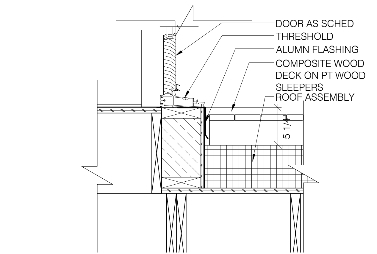
8 SILL - ROOFTOP DOOR SCALE: 1-1/2" = 1'-0"
