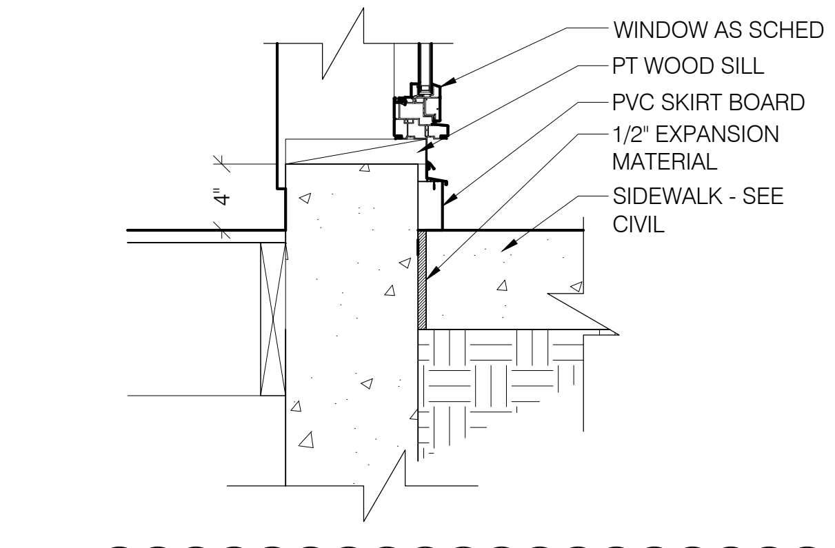
10 SILL - FRONT SIDE LIGHTS SCALE: 1-1/2" = 1'-0"
