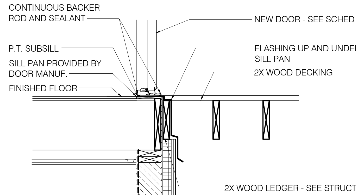
5 DECK DETAIL SCALE: 1" = 1'-0"
