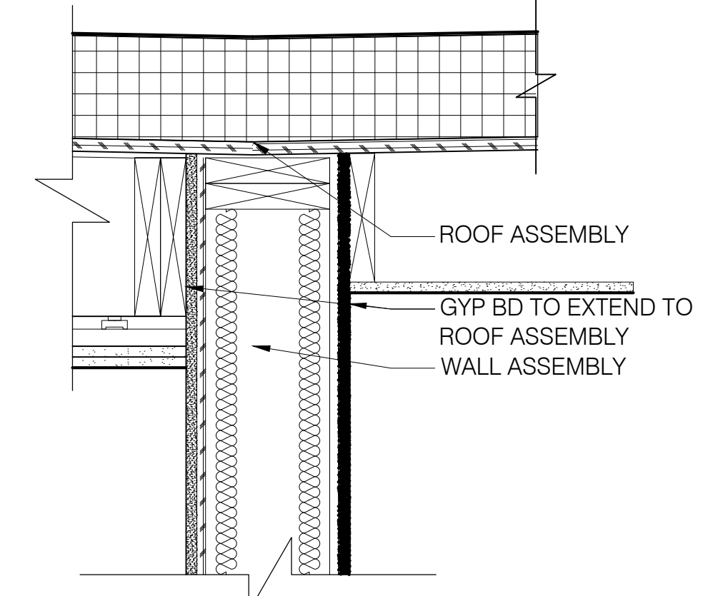
11 T.O. WALL @ STAIR SHAFT SCALE: 1-1/2" = 1'-0"
