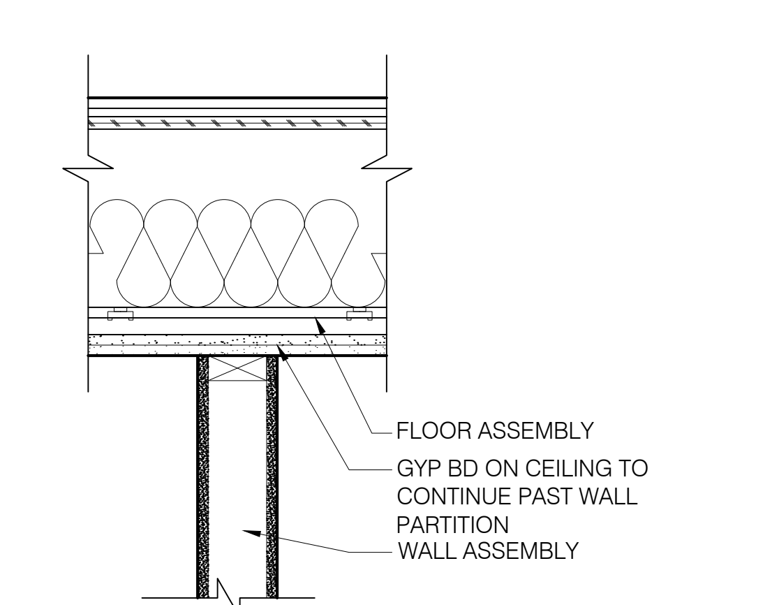
13 T.O. PARTITION SCALE: 1-1/2" = 1'-0"
