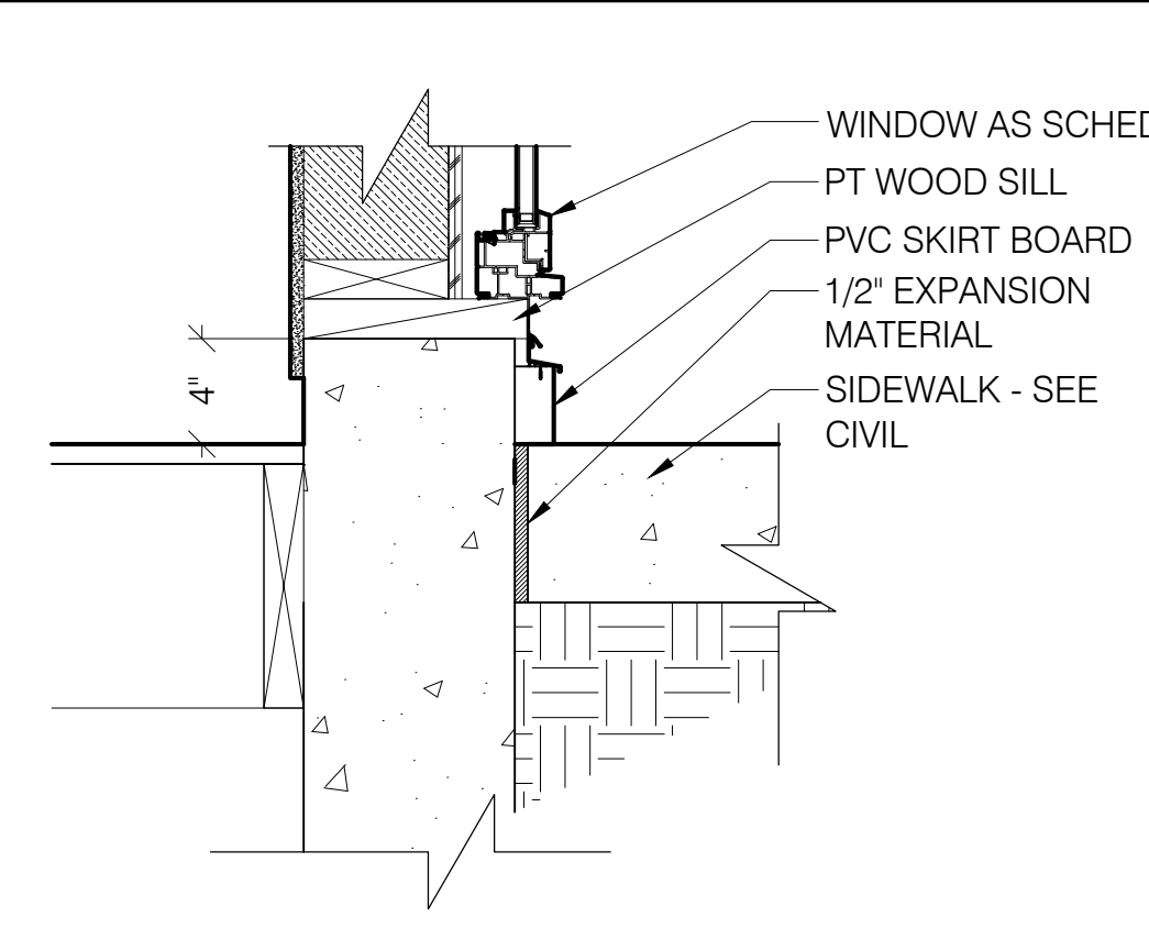
10 SILL - FRONT SIDE LIGHTS SCALE: 1-1/2" = 1'-0"
