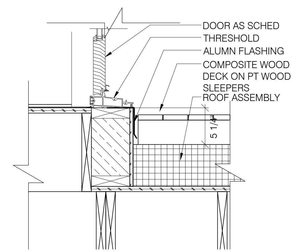
8 SILL - ROOFTOP DOOR SCALE: 1-1/2" = 1'-0"
