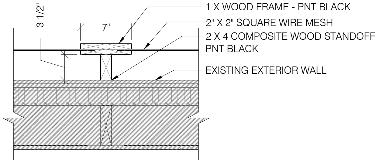
2 DETAIL SECTION 0 4" SCALE: 1'-1/2" = 1'-0"
