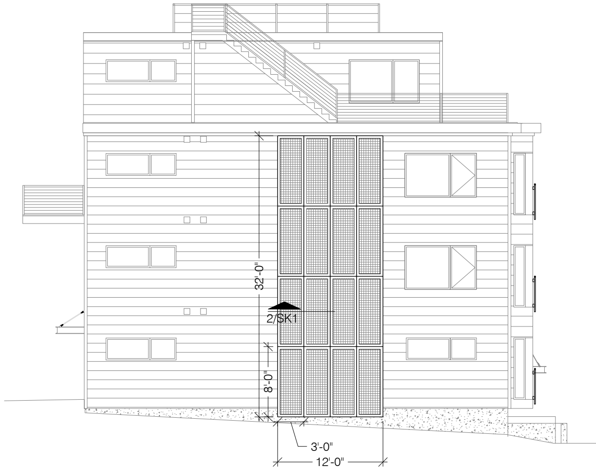
1 SCREEN ELEVATION 0 5'-4" SCALE: 3'-32" = 1'-0"
