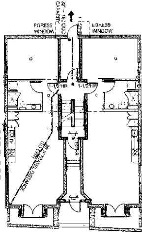
FIRST FLOOR SCALE: 1/8" = 1'-0"
