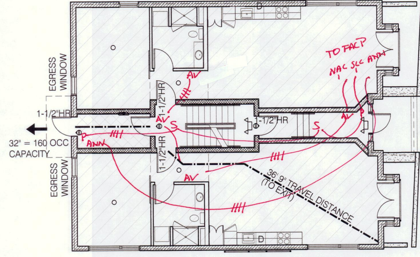
2 FIRST FLOOR SCALE: 1/8" = 1'-0"
