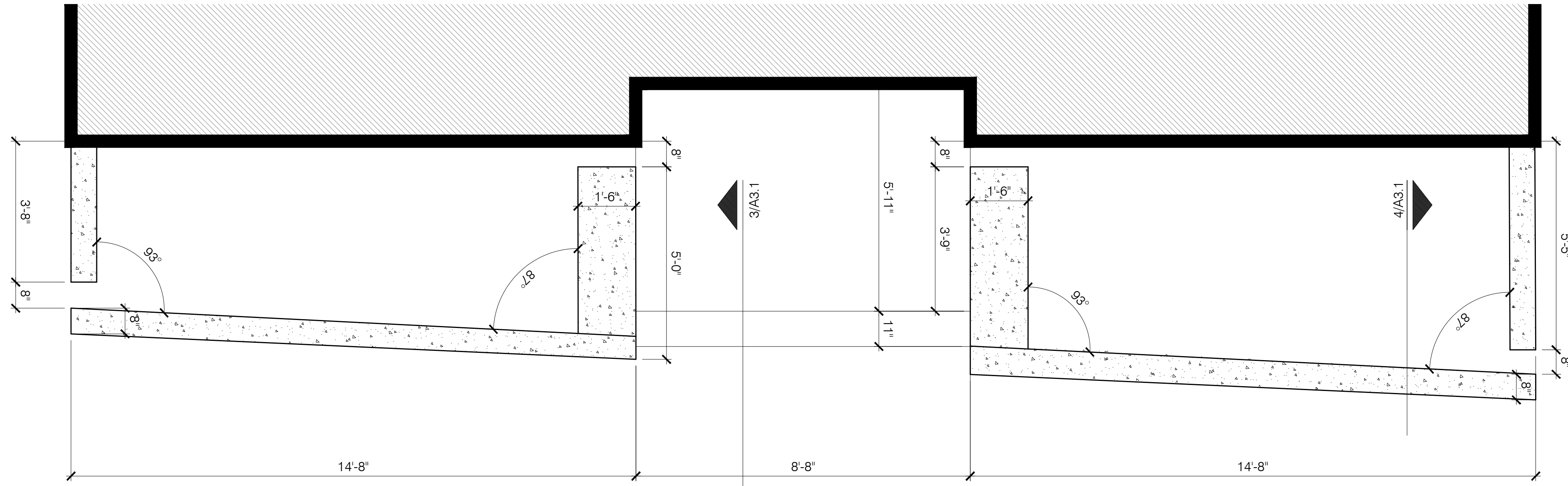
3 PLANTER SCALE: 1/4" = 1'-0"
