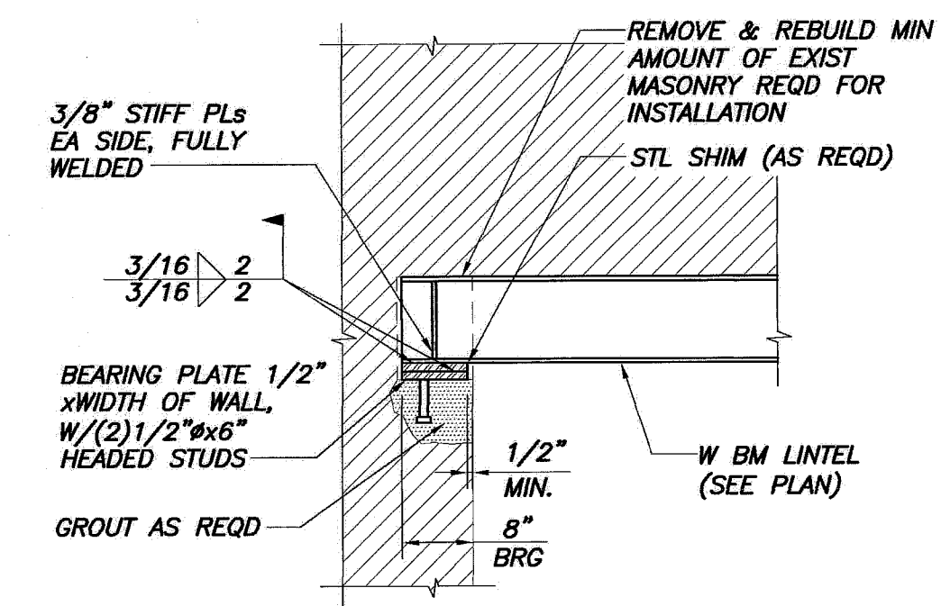
TYP BEAM POCKET DETAIL U.N.O. N.T.S.
