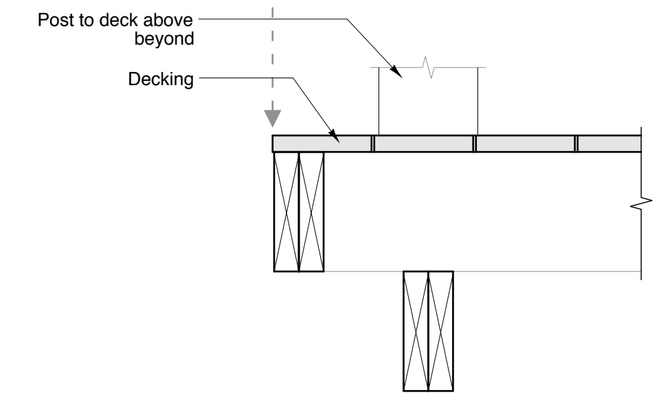
5 Edge of Deck Detail SCALE: 1 1/2" = 1'-0"
