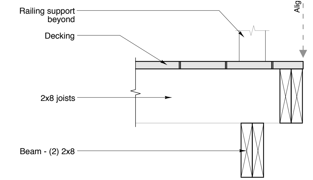
2 Edge of Deck Detail SCALE: 1 1/2" = 1'-0"
