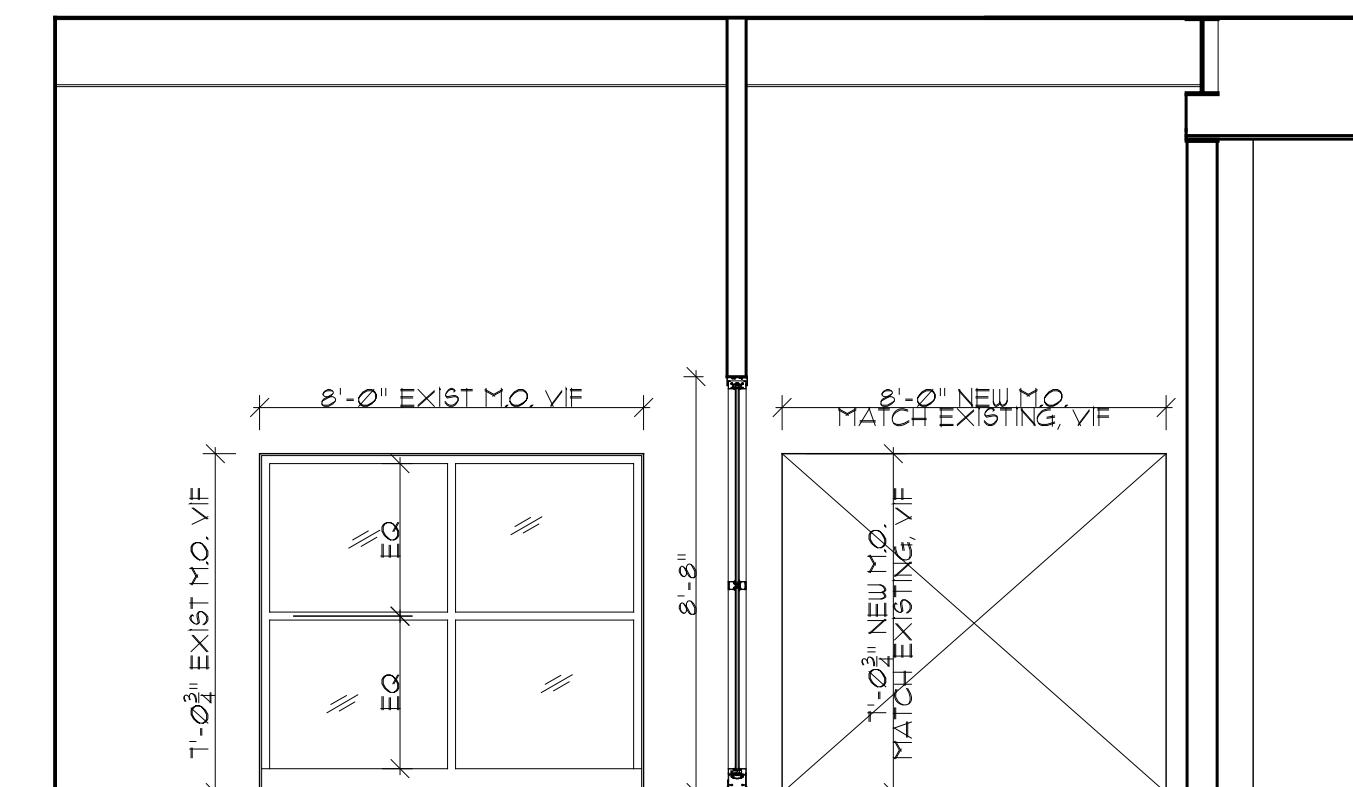
4 SECTION 5 A302 SCALE: 1/4"=1'-0"
