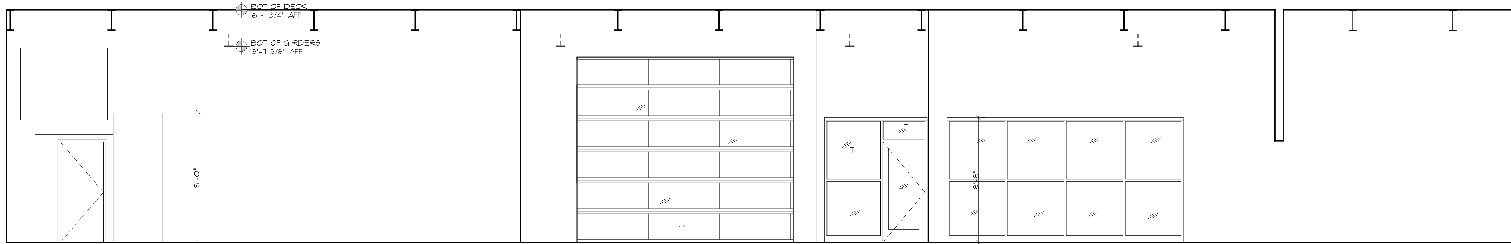
2 SECTION 3 A302 SCALE: 1/4"=1'-0"
