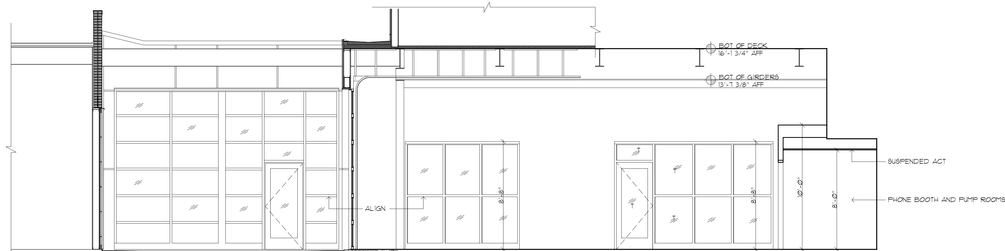
3 SECTION 4 A302 SCALE: 1/4"=1'-0"
