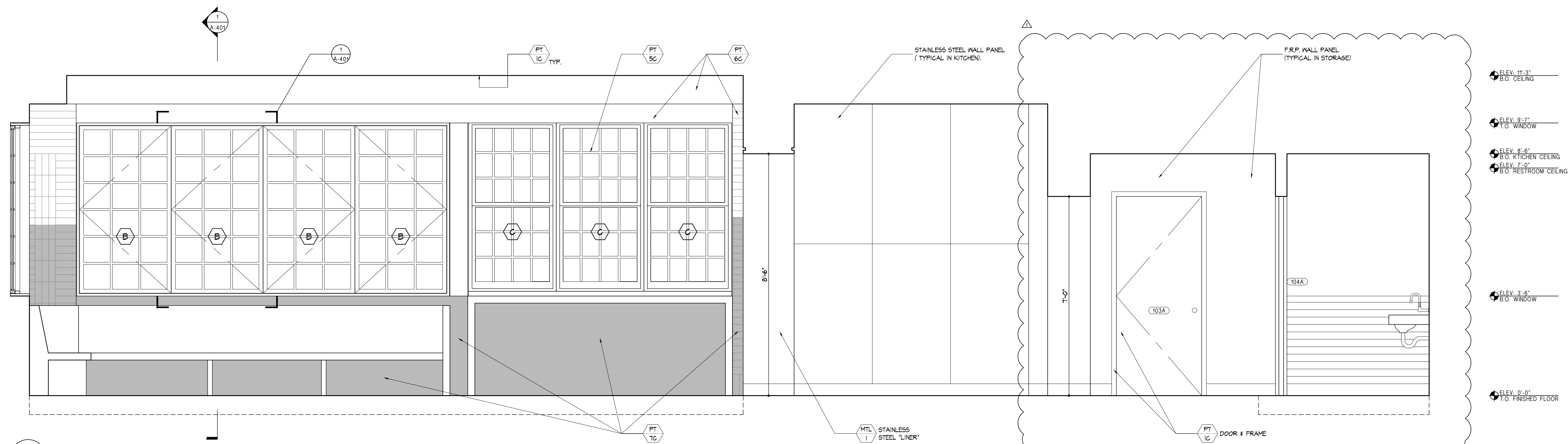
1 Section Scale: 1/2" = 1'-0"
