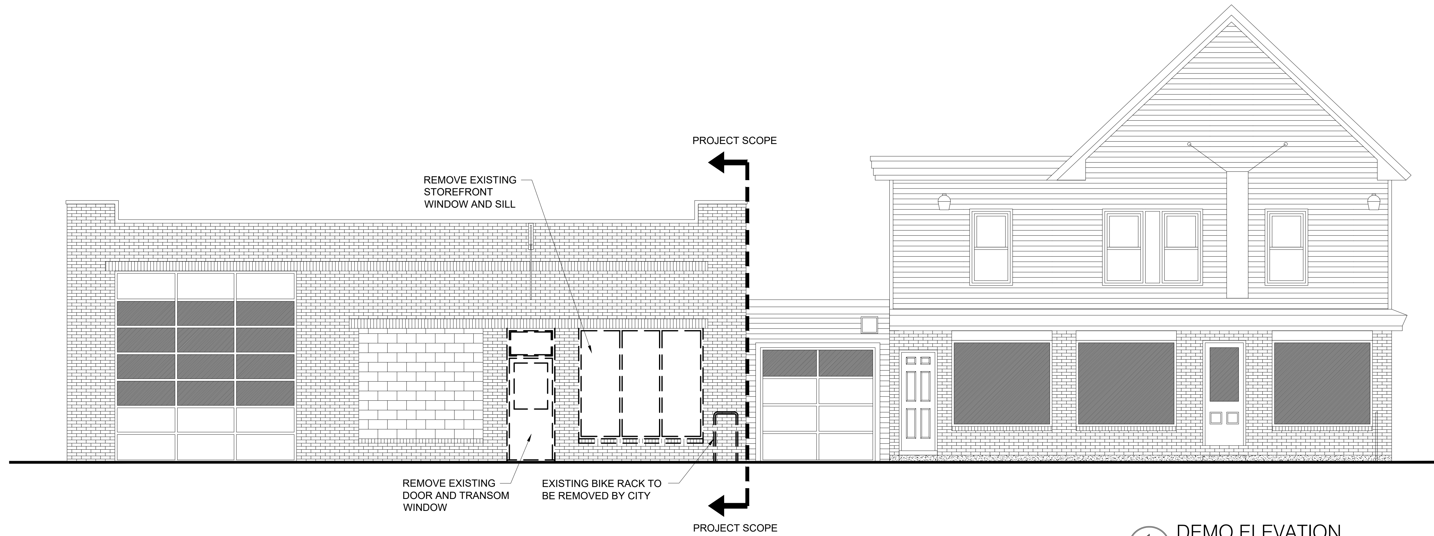
1 DEMO ELEVATION SCALE: 1/4" = 1'-0"
