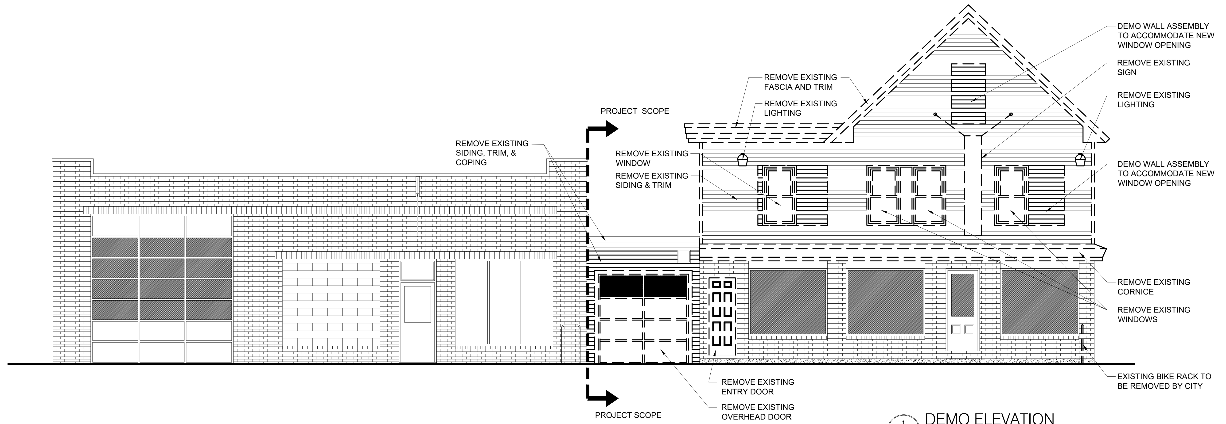
1 DEMO ELEVATION SCALE: 1/4" = 1'-0"
