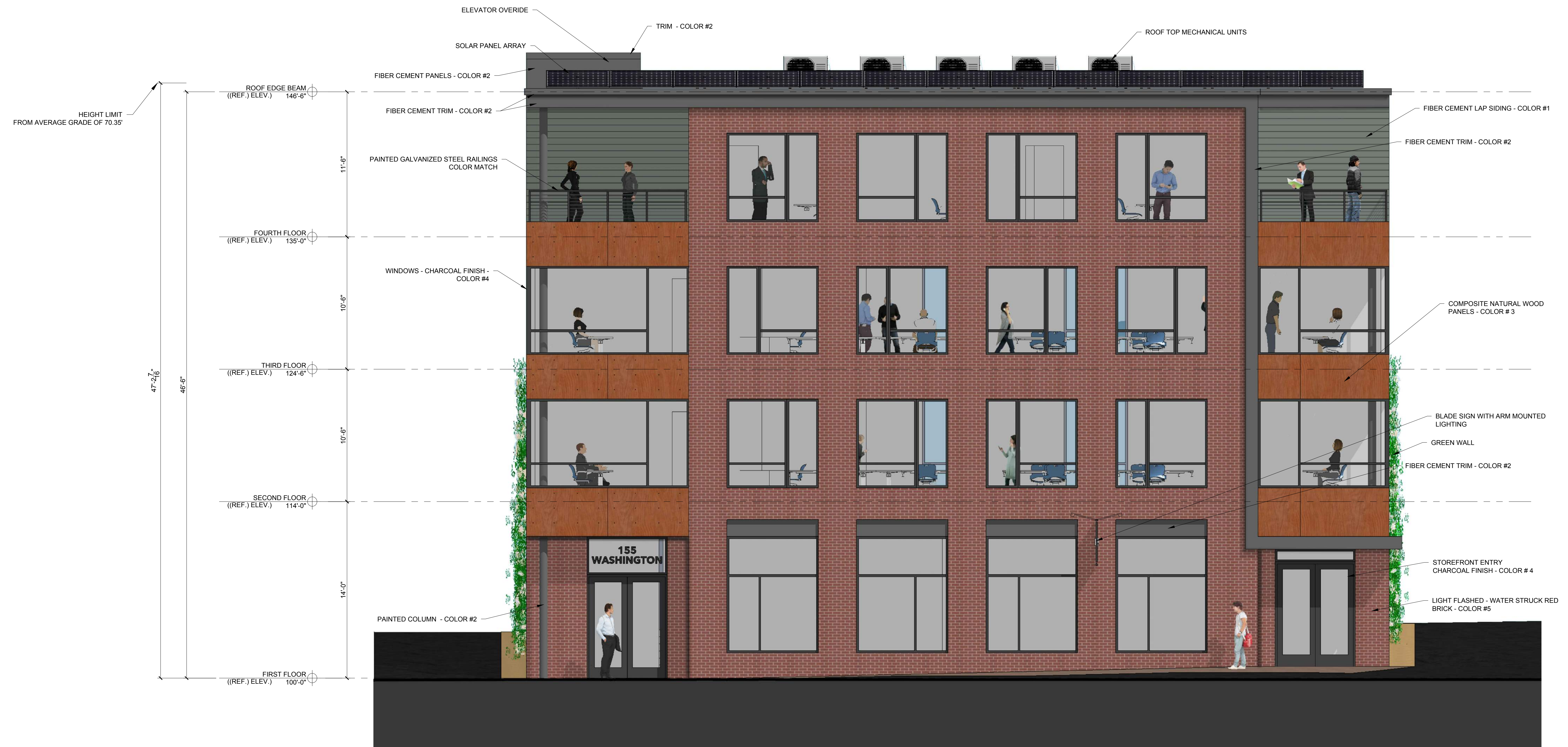
1 WEST EXTERIOR ELEVATION N.T.S.
