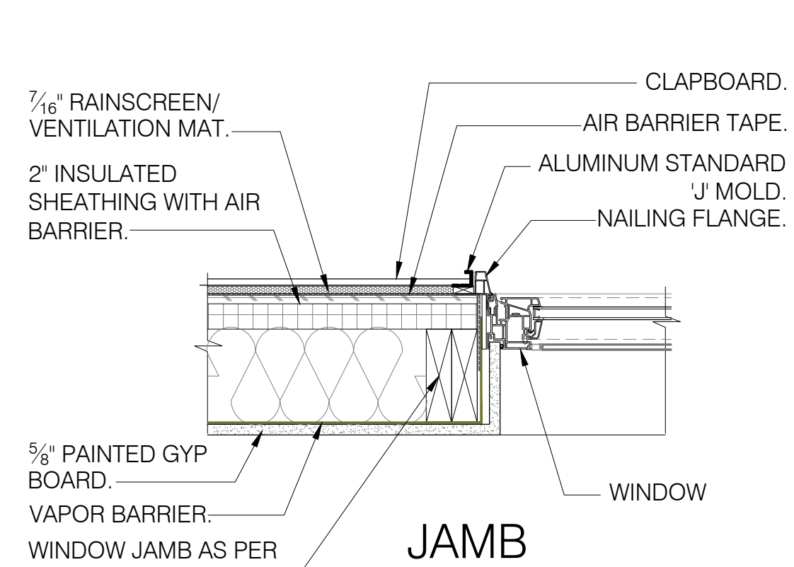
2 WINDOW DTLS - TYP. SCALE: 1-1/2" = 1'-0"
