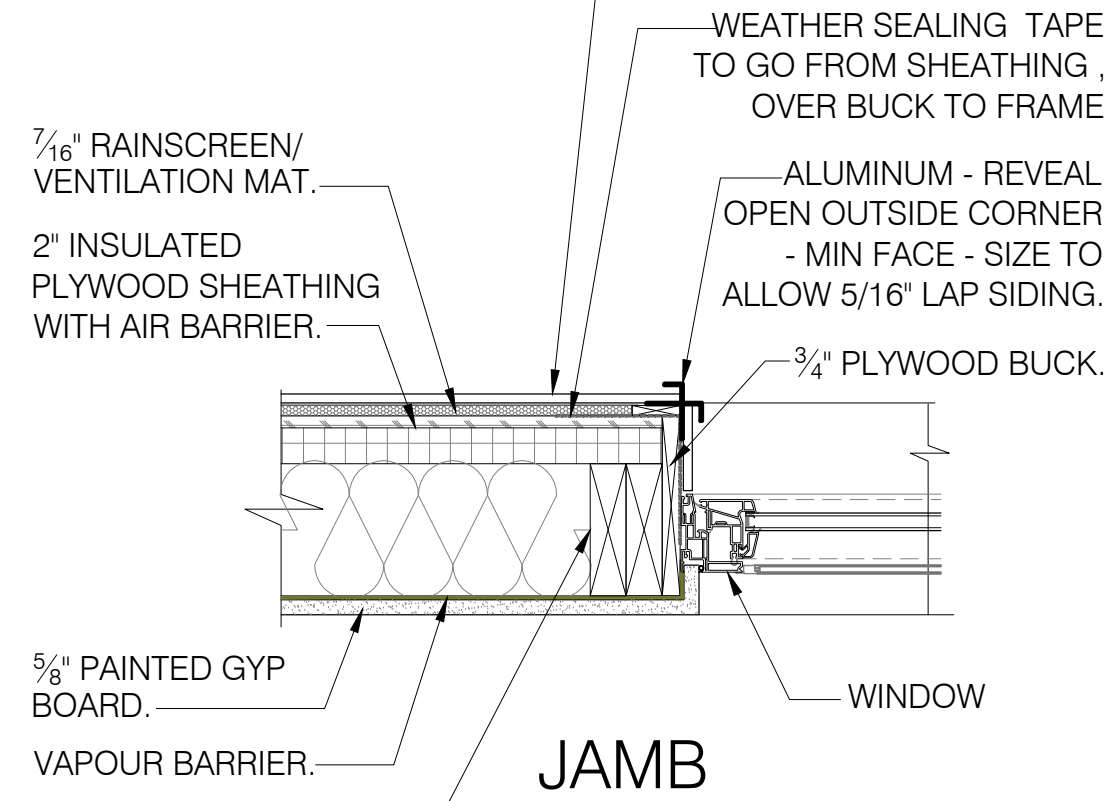
1 WINDOW DTLS - TYP. SCALE: 1-1/2" = 1'-0"
