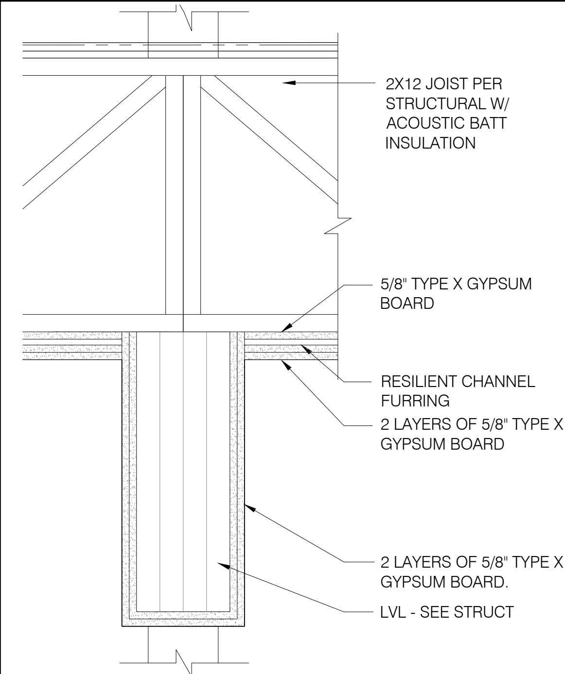
9 LVL WRAP DETAIL SCALE: 1 1/2" = 1'-0"
