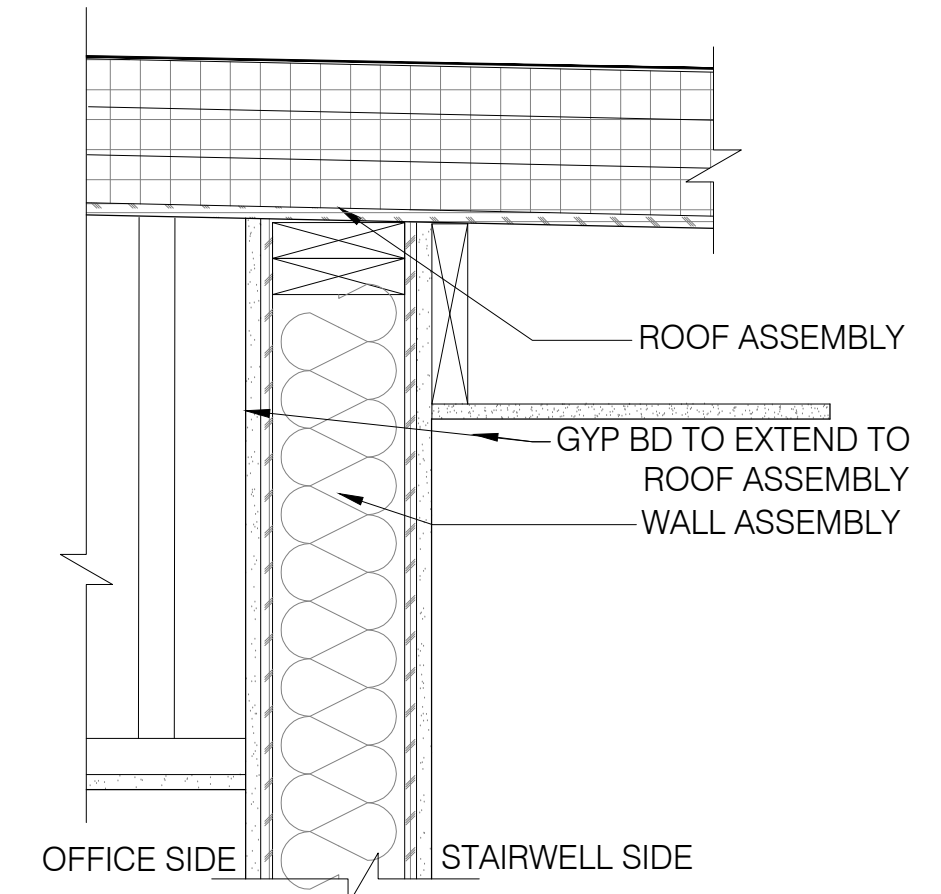
5 T.O. WALL @ STAIR SHAFT SCALE: 1 1/2" = 1'-0"
