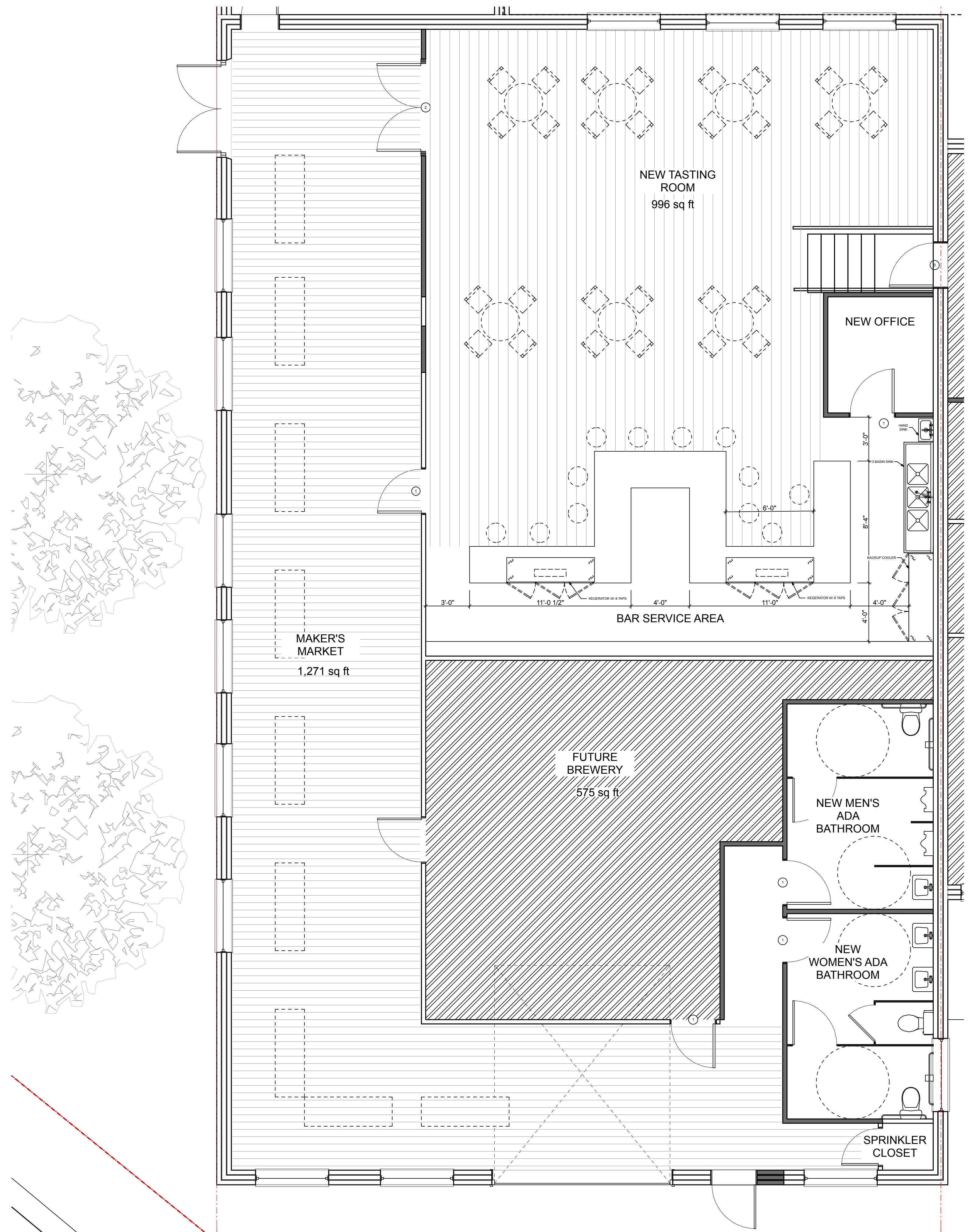
1 MAIN LEVEL SCALE: 1/4" = 1'-0"
