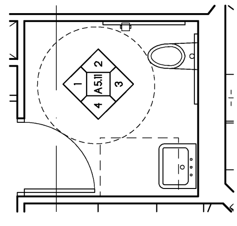
J W.C. 305 SCALE: 1/4" = 1'-0"
