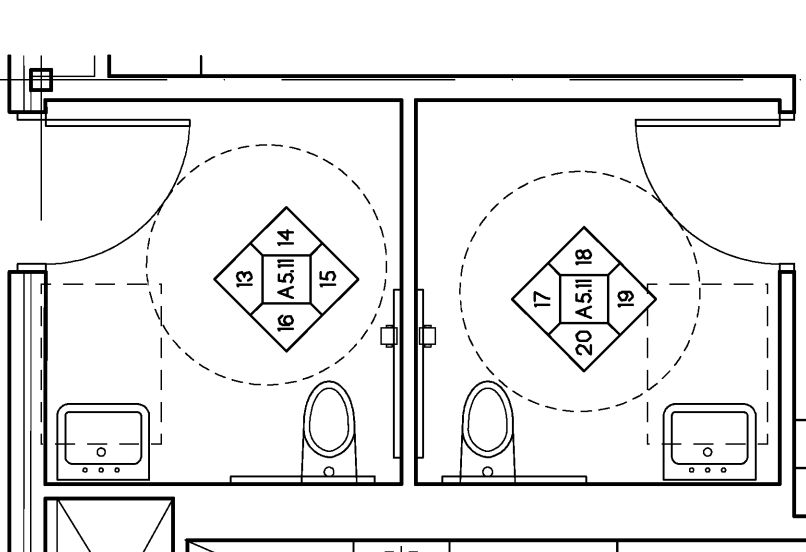
M W.C. 228, 242, 255 SCALE: 1/4" = 1'-0"
