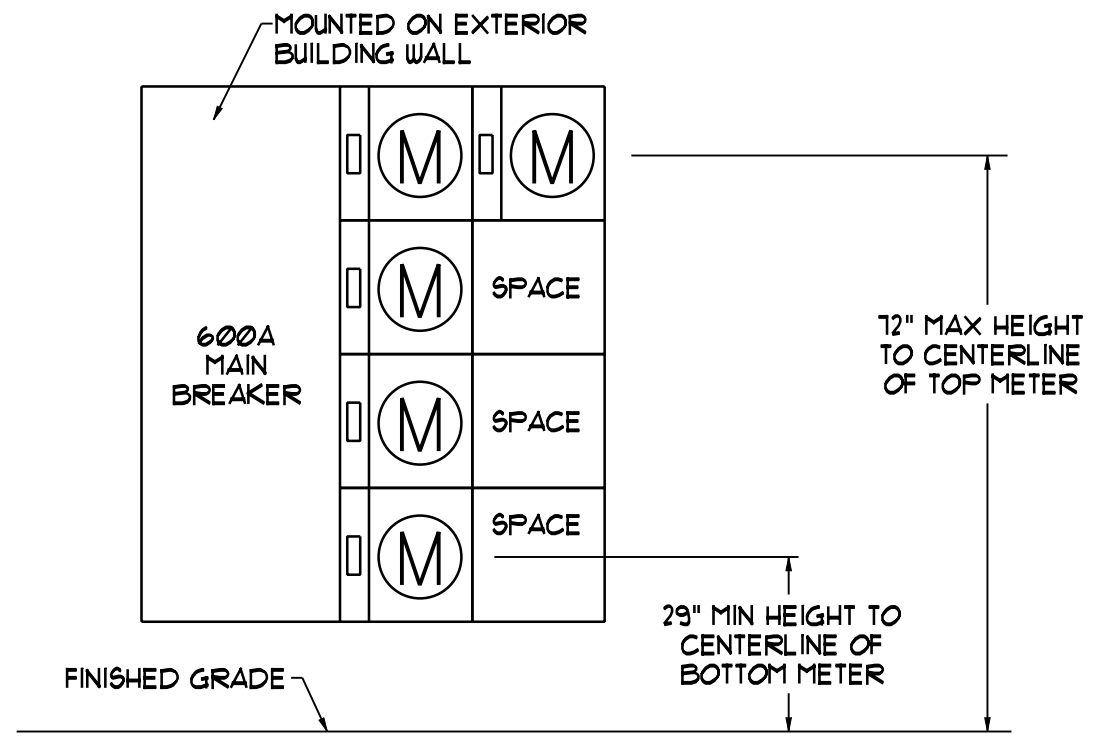
METER STACK ELEVATION - (BUILDING 'C') SCALE: NONE
