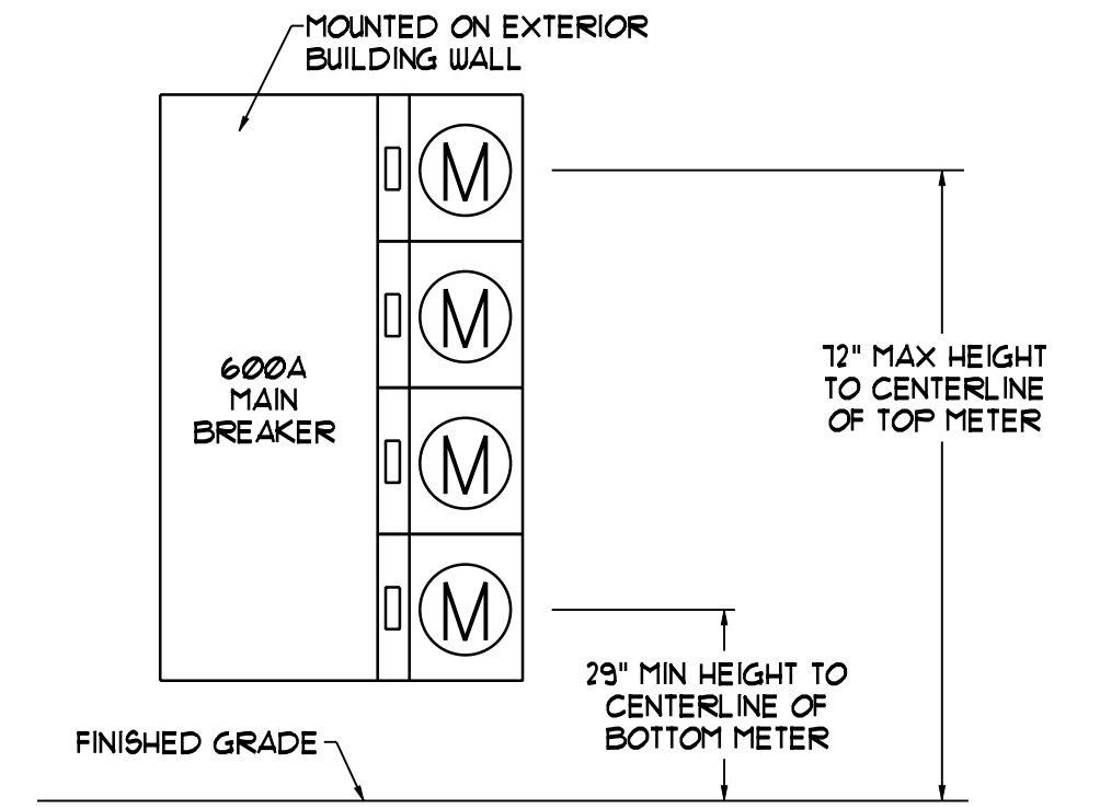
METER STACK ELEVATION - (BUILDINGS 'A', 'B' & 'D') SCALE: NONE
