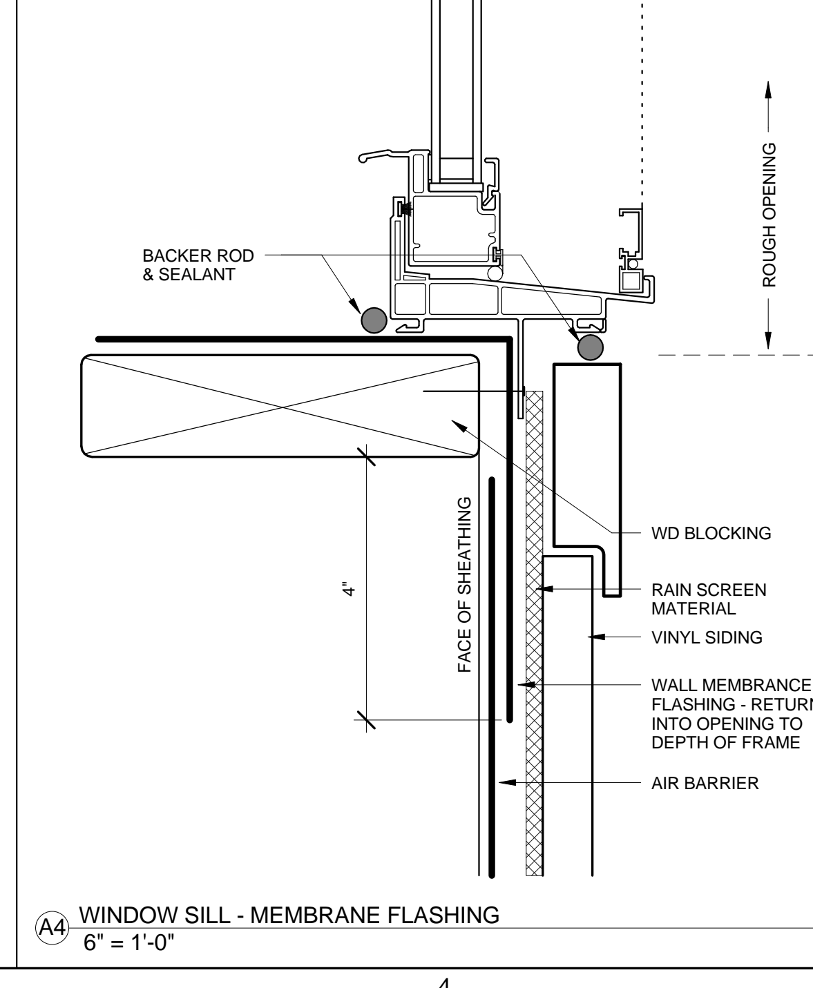
A4 WINDOW SILL - MEMBRANE FLASHING 6" = 1'-0"
