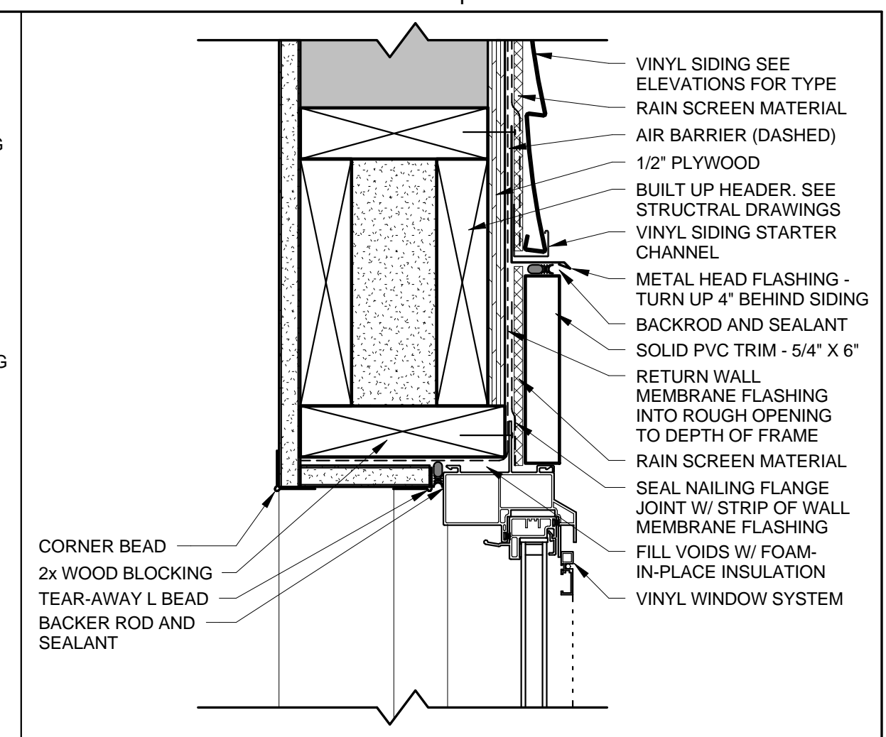
D1 WINDOW HEAD DETAIL 3" = 1'-0"
