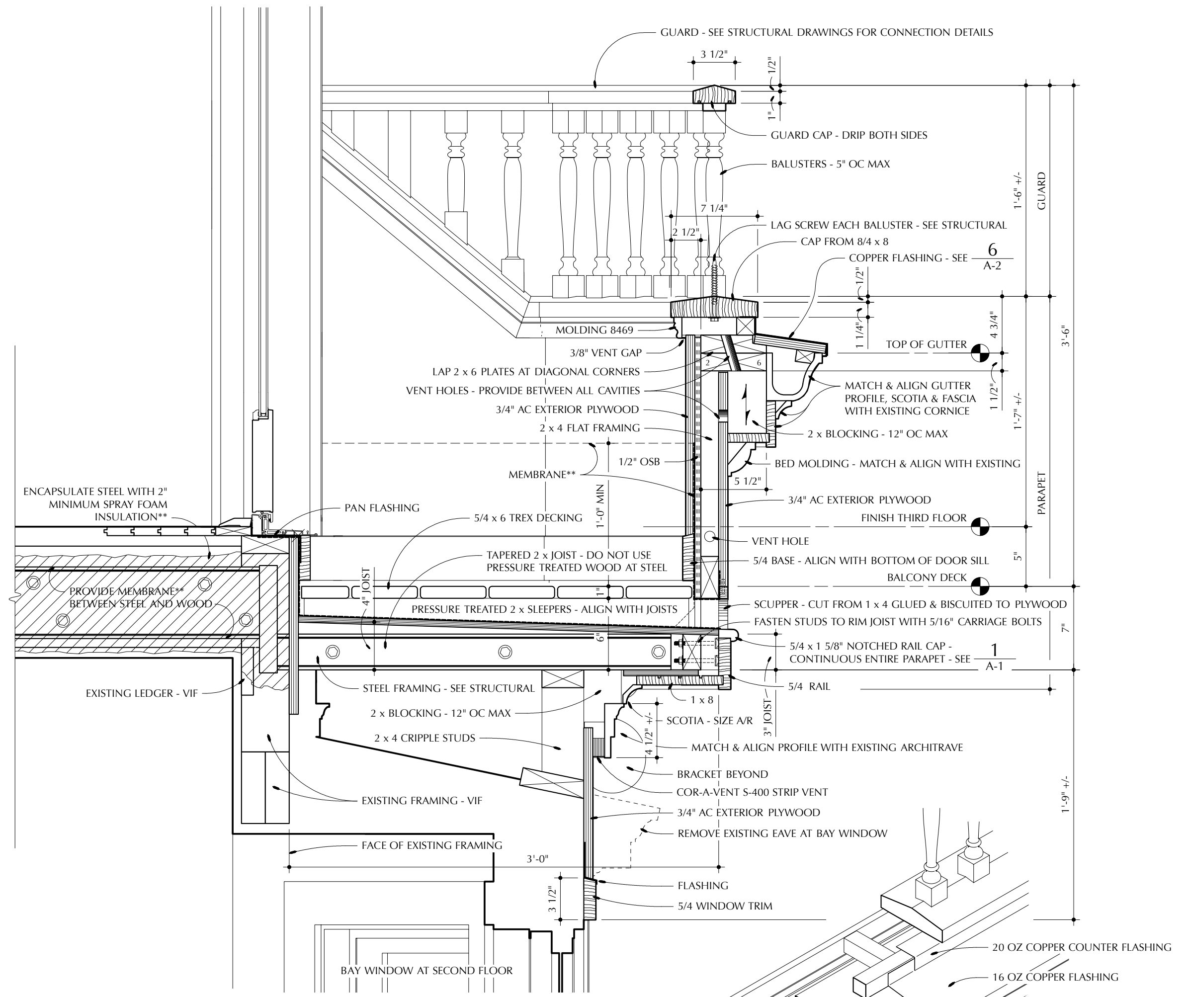
2 CROSS SECTION Scale: 1 1/2" = 1'-0"
