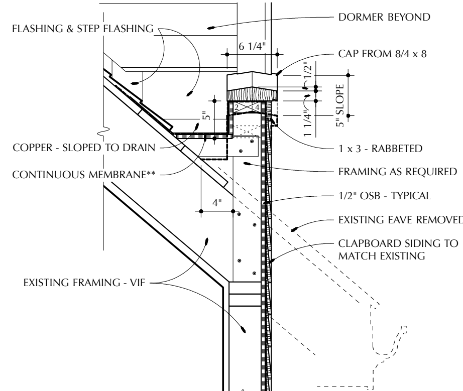
4 SECTION AT DIVERTER Scale: 1" = 1'-0"
