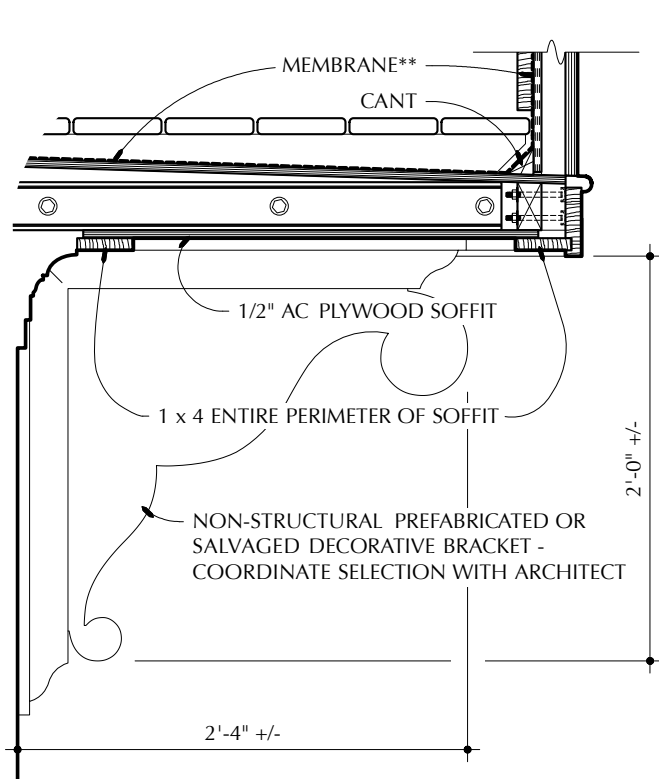
3 DECORATIVE BRACKET Scale: 1" = 1'-0"
