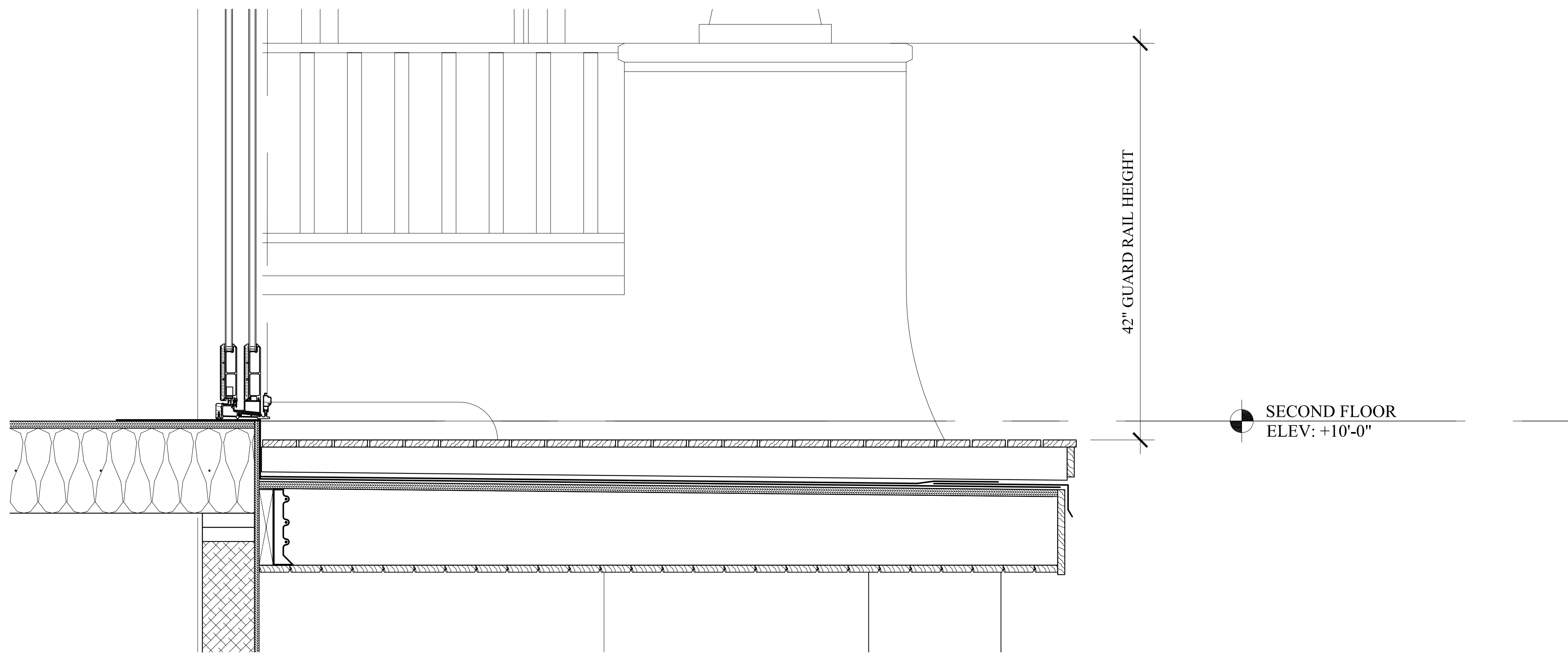
DD3 DECK DETAIL A-3.2 SCALE: 1 1/2" = 1'-0"
