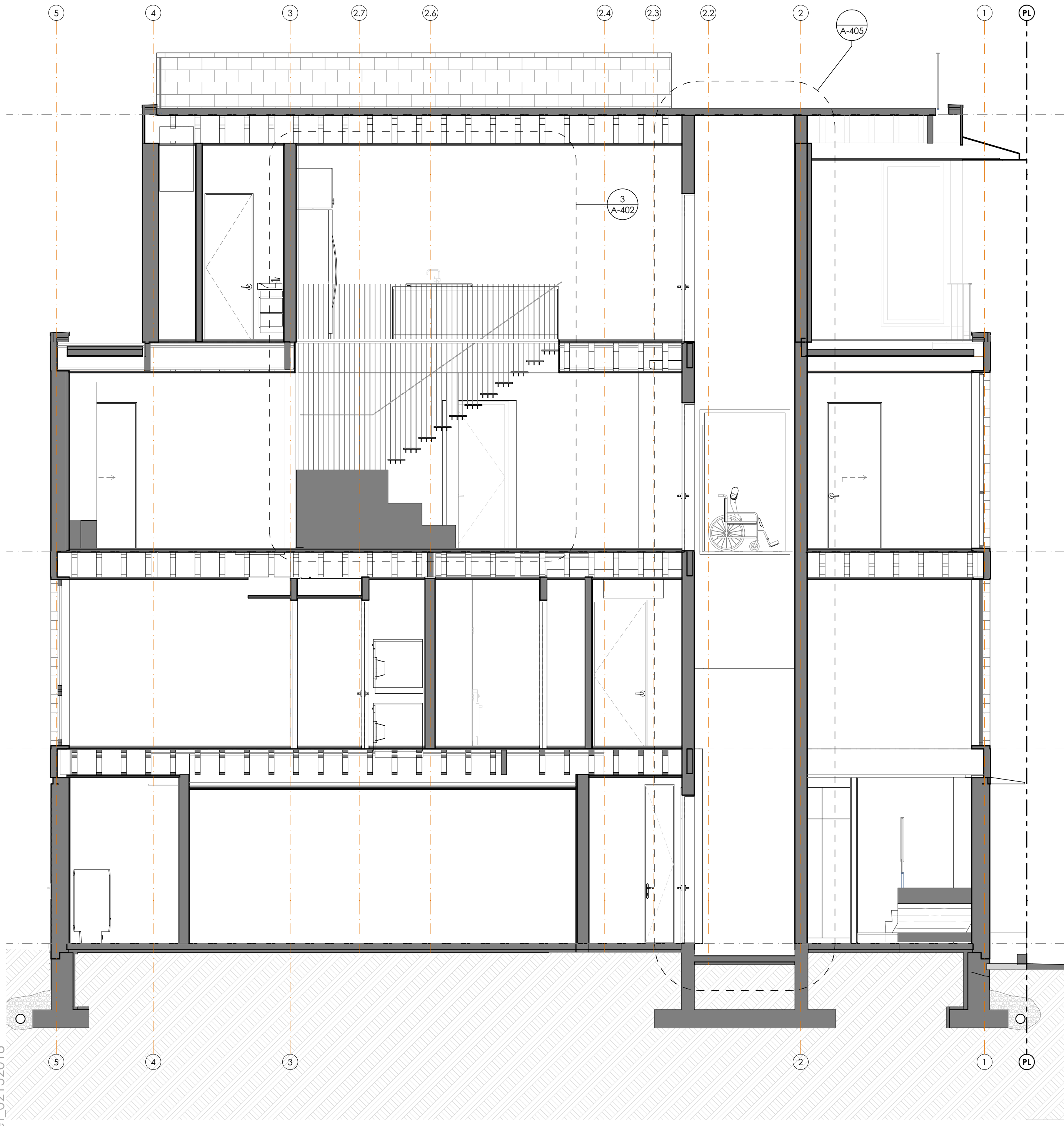
2 BUILDING SECTION - LONGITUDINAL 3 SCALE: 1/4" = 1'-0"
