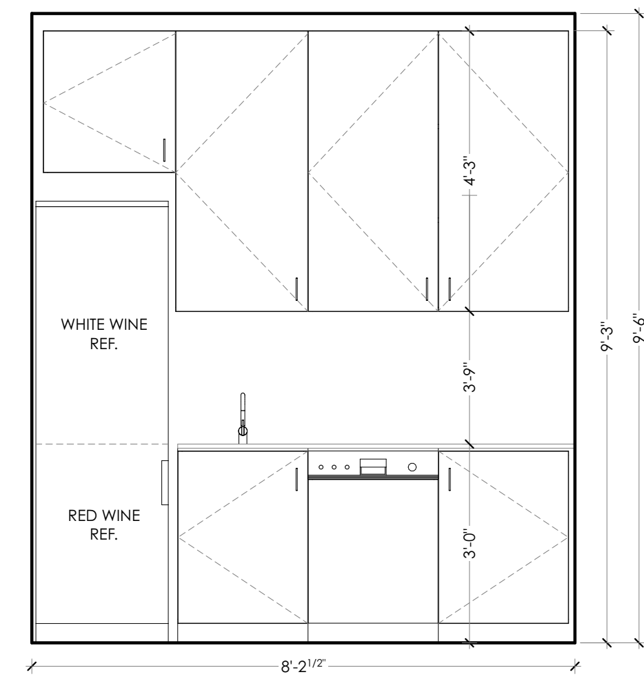
4 PANTRY SCALE: 1/2" = 1'-0"
