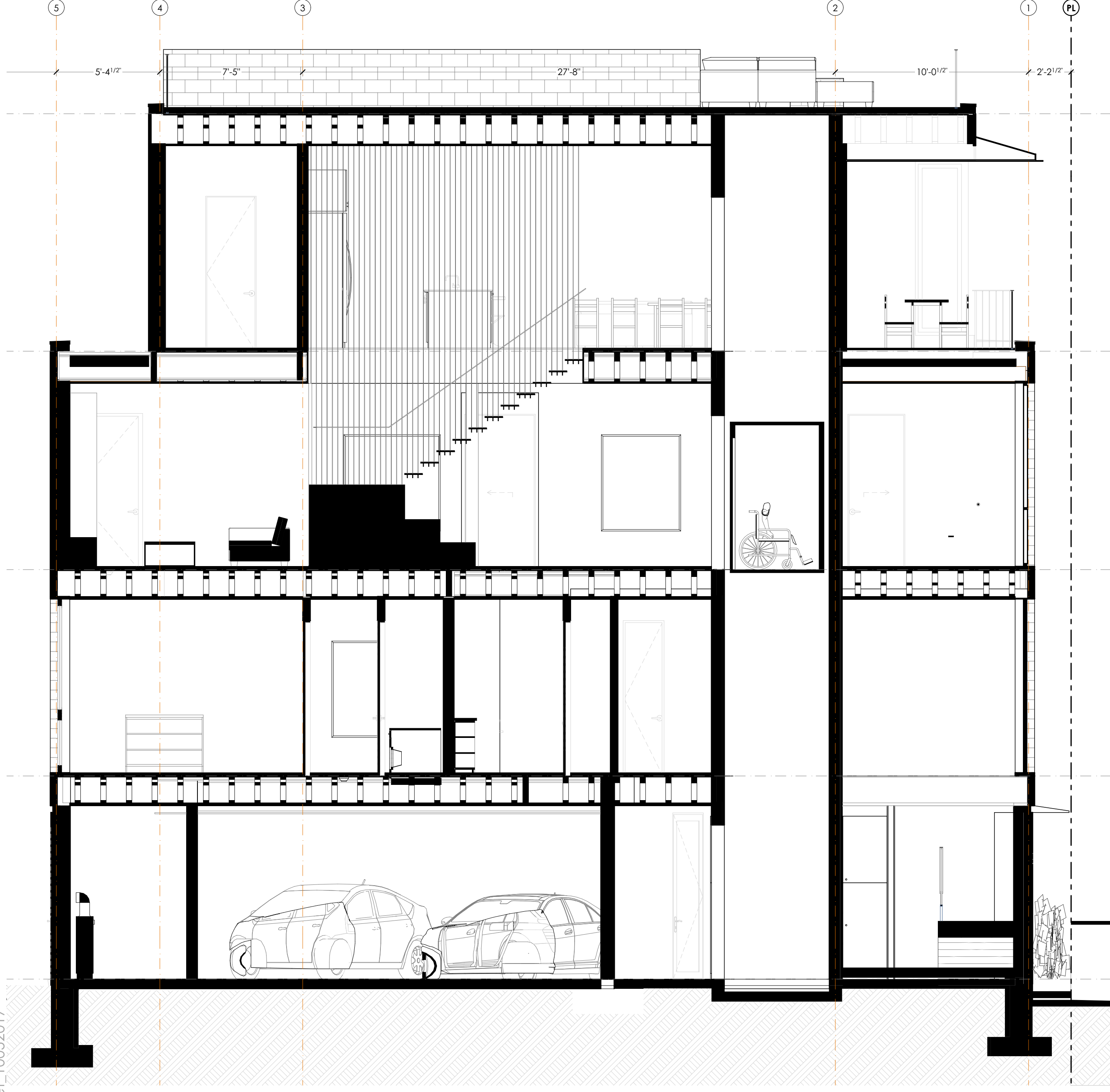
2 BUILDING SECTION - LONGITUDINAL 3 SCALE: 1/4" = 1'-0"
