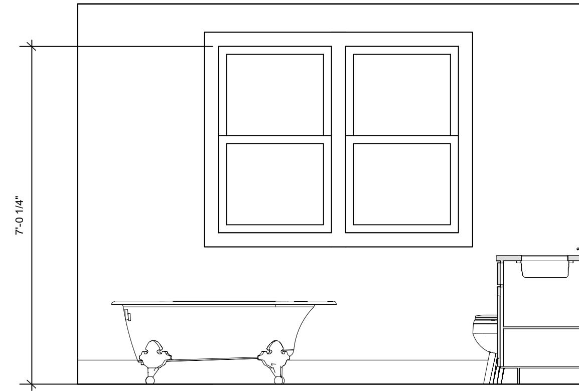
3 MASTER BATH TUB Scale: 1/2" = 1'-0"
